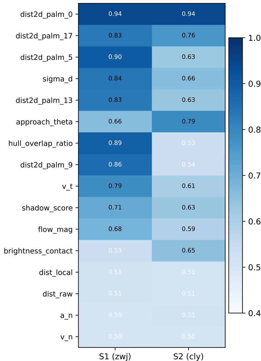
(b) Exp-A AUROC
