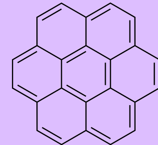
Coronene
