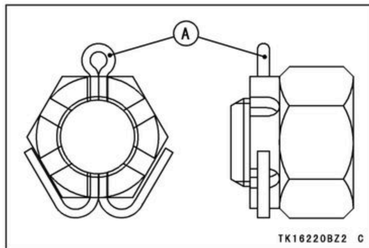
A. Cotter Pin
