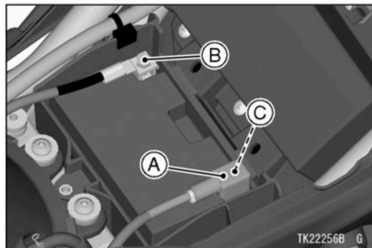
A. Red Cap B. (–) Terminal C. (+) Terminal
