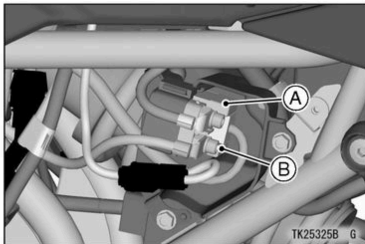
A. Main Fuse 30 A B. Spare Fuse 30 A
