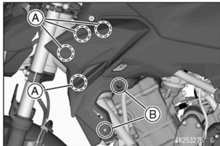
A. Quick Rivets B. Bolts
