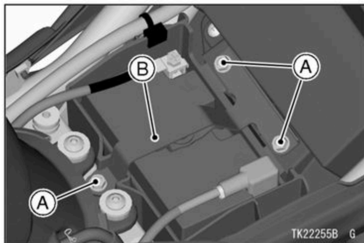
A. Bolts B. Holder
