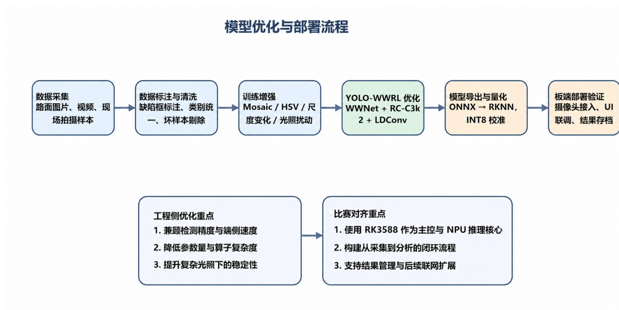
图 1 模型优化与板端部署流程
