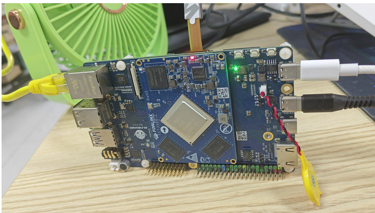
图 3 RK3588（ELF 2）开发板实物
