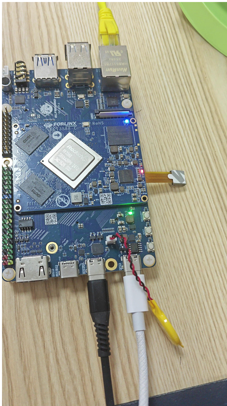
图 4 摄像头与开发板 MIPI 接入细节
