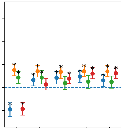
MMTC
