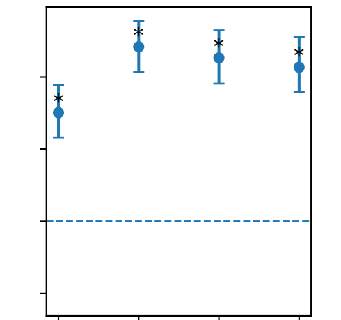
MMTC
