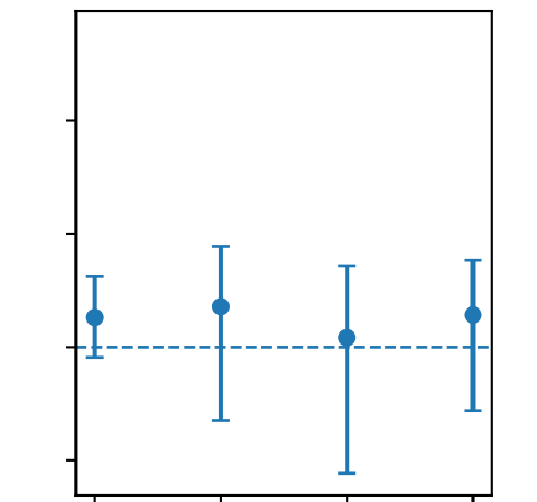
PFSMB
