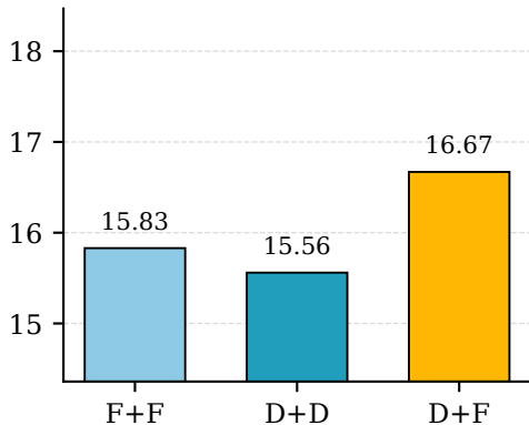
HMMT 2025
