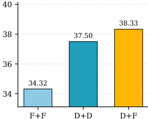
AIME 2025
