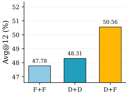
AIME 2024
