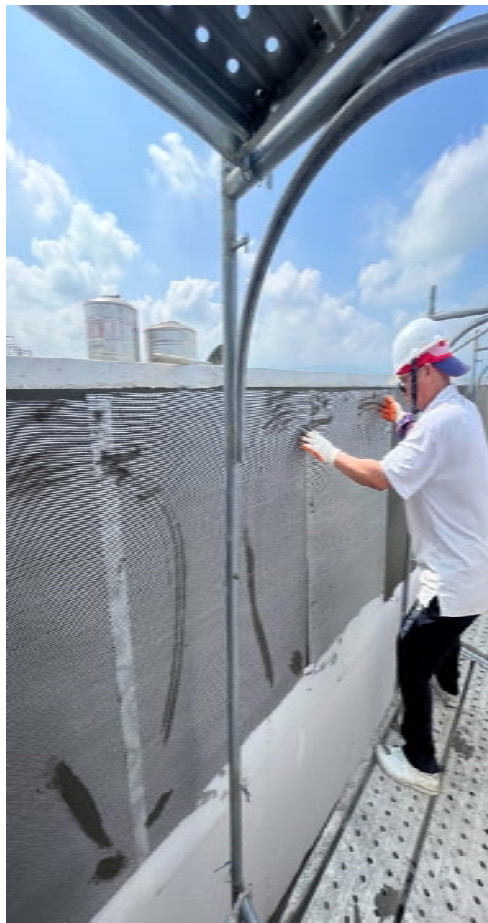
抗拉玻纖網安裝
