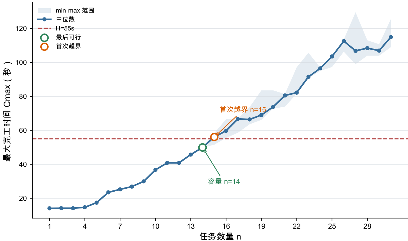
固定 4 台 AMR 下的任务负荷容量边界
