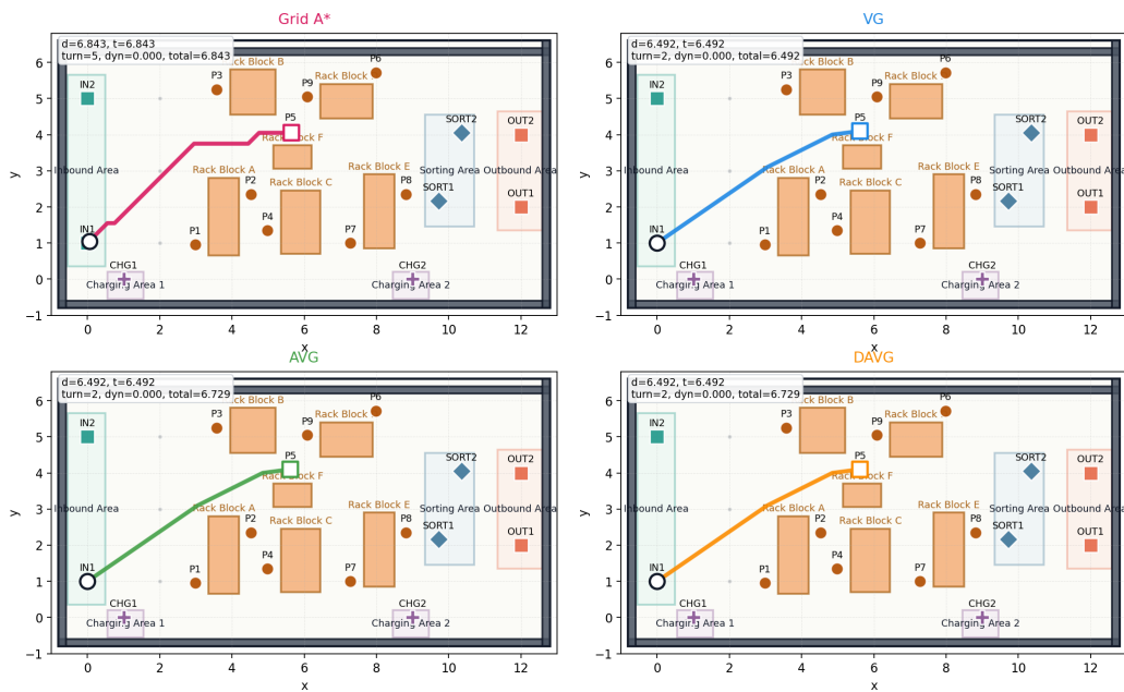
图 2: IN1 → P5 的四类 P1 路径形态对比
