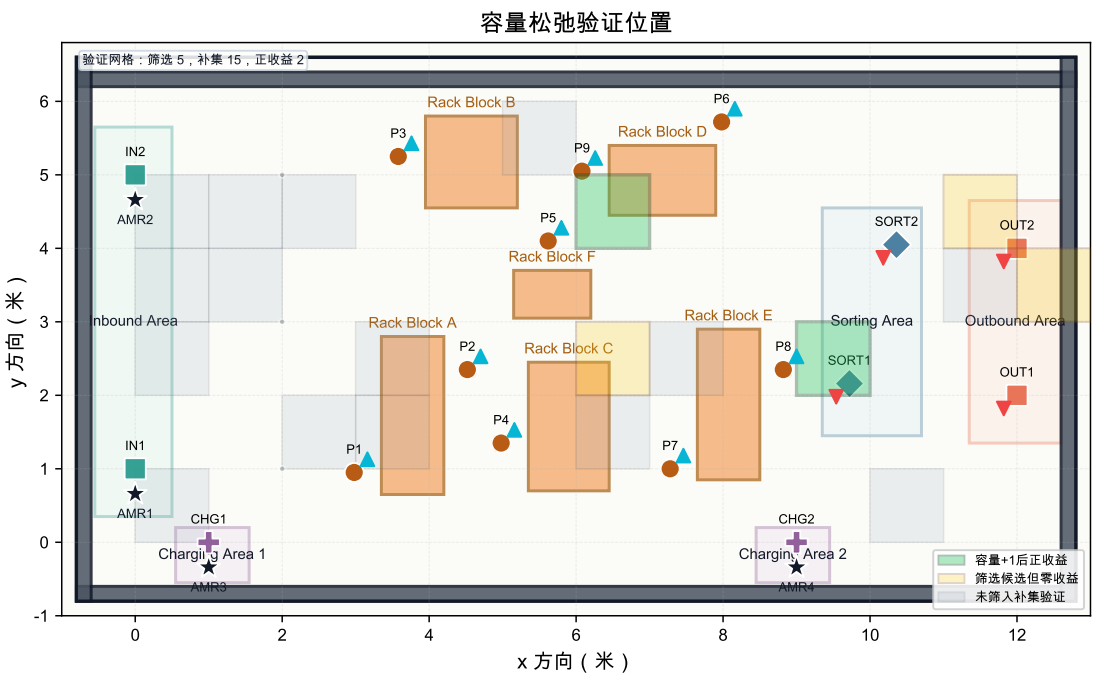
图 7: 瓶颈空间簇容量松弛验证位置
