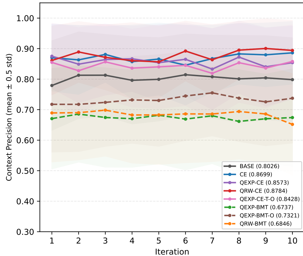
Context Precision
