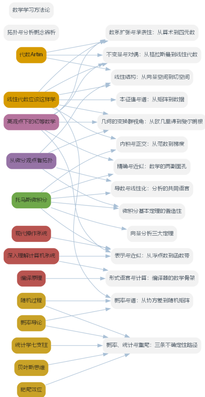
图 3 书与交叉主线：左侧为已收录教材，右侧为把它们缝在一起的桥接主题页。一张图就能看出哪些书是「孤岛」、哪些书已被主线串起来。
