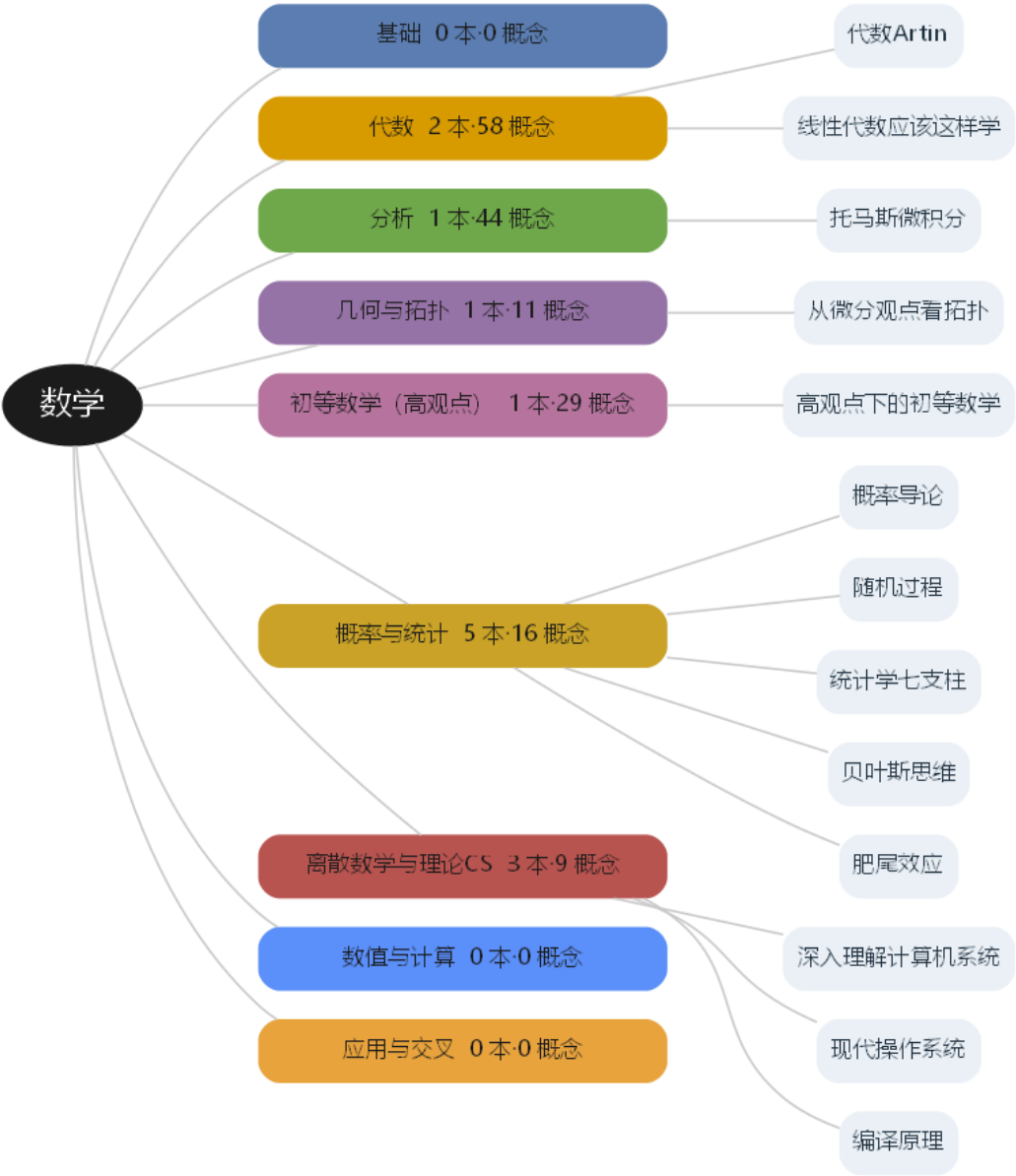
图 2 分支与书目：从「数学」出发，按九个分支组织。每个分支标注已收录书籍数与概念节点数；叶子节点是具体的书。
