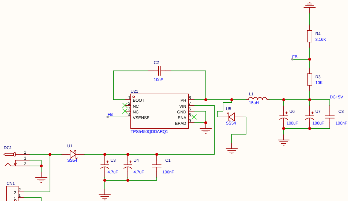
DCDC电路
