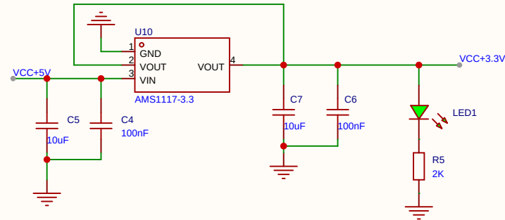
LDO电路
