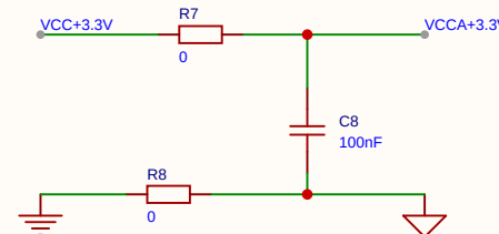
模数地隔离
