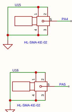
DAC接口
