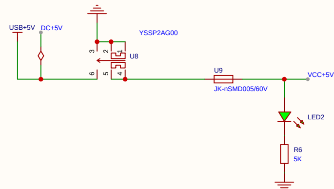
电源合路
