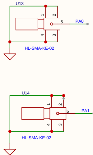
ADC接口
