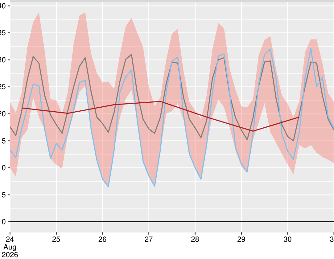
Кърджали (15730), 2026-08-30 06:00:00
