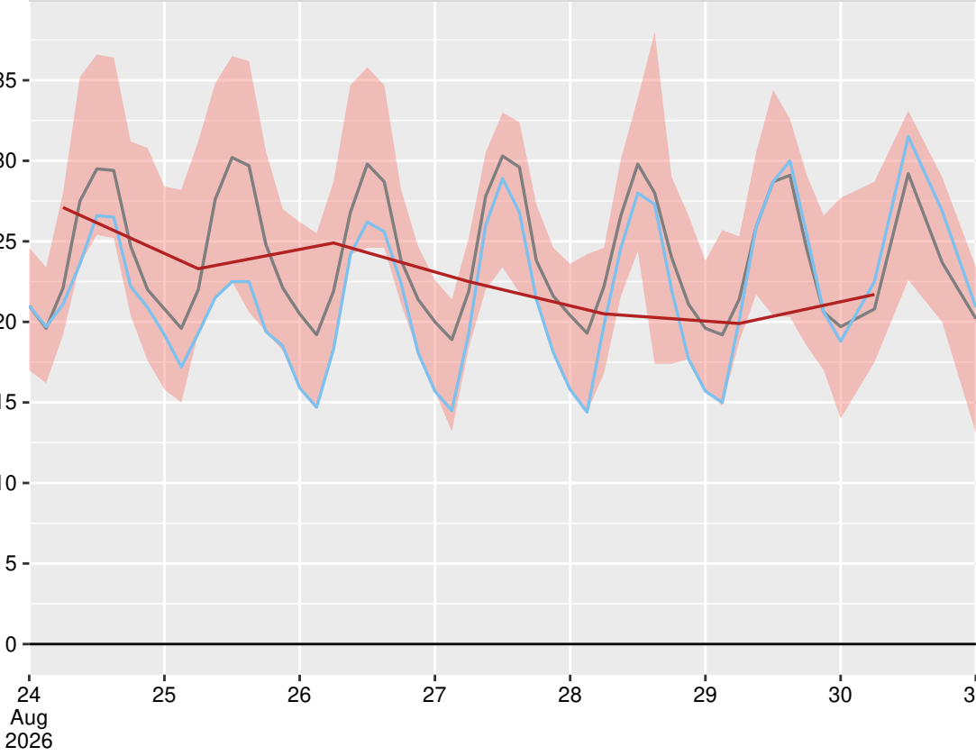
Сливен (15640), 2026-08-30 06:00:00
