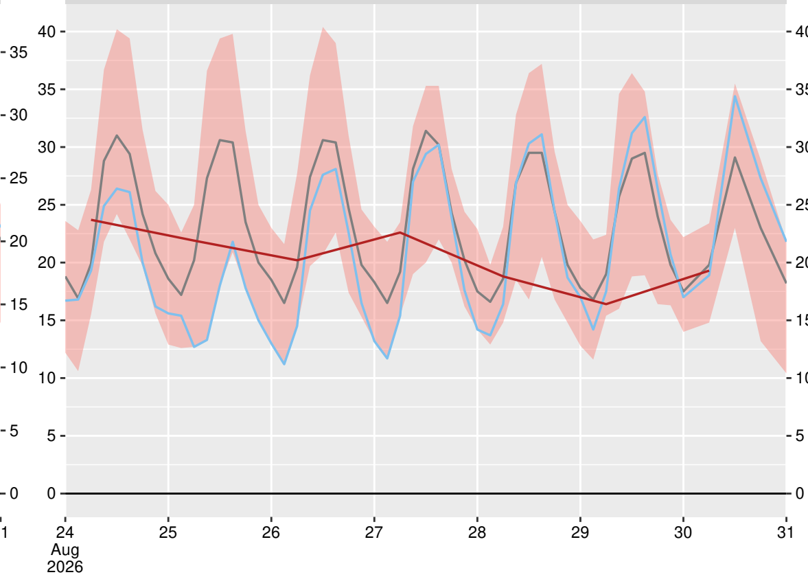
Сандански (15712), 2026-08-30 06:00:00
