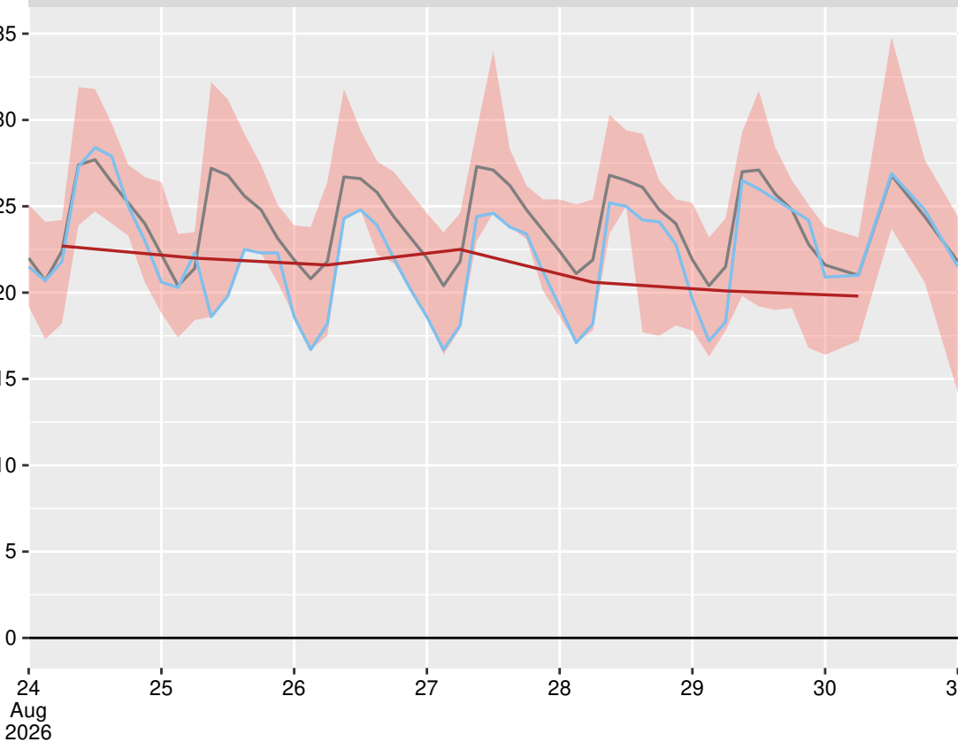
Видин (15502), 2026-08-30 06:00:00
