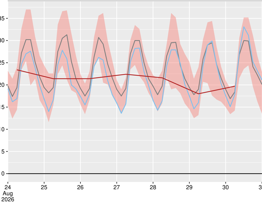
Разград (15549), 2026-08-30 06:00:00
