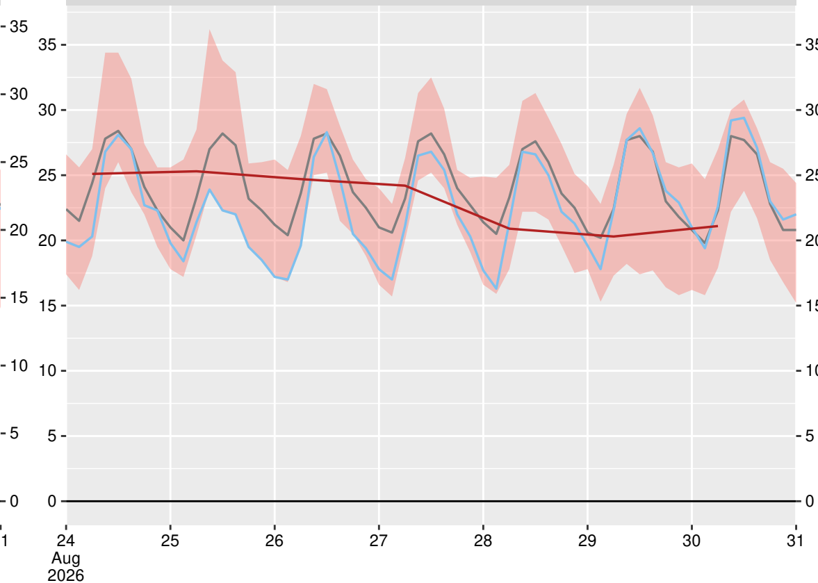
вр. Мусала (15615), 2026-08-30 06:00:00
