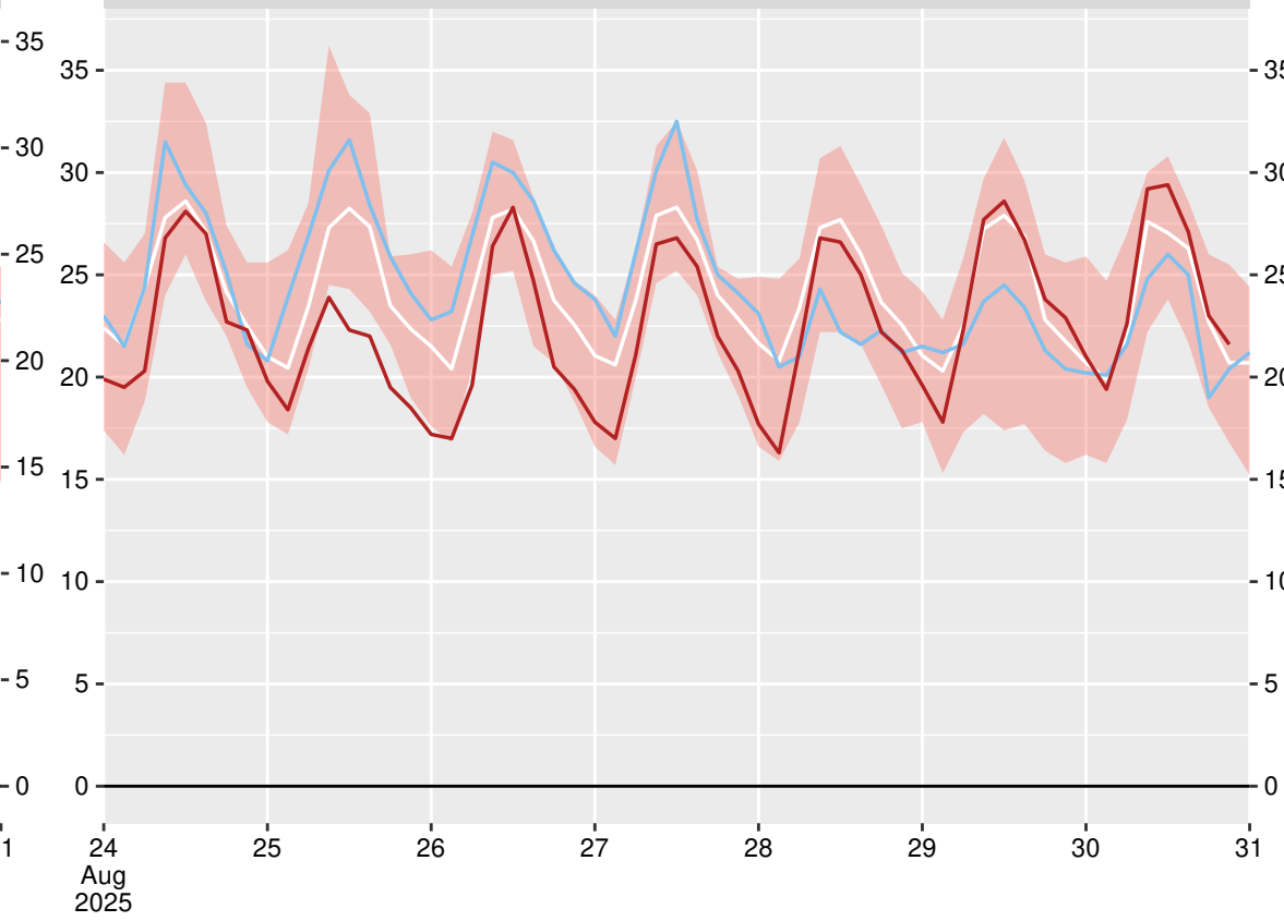
вр. Мусала (15615), 2025-08-30 21:00:00
