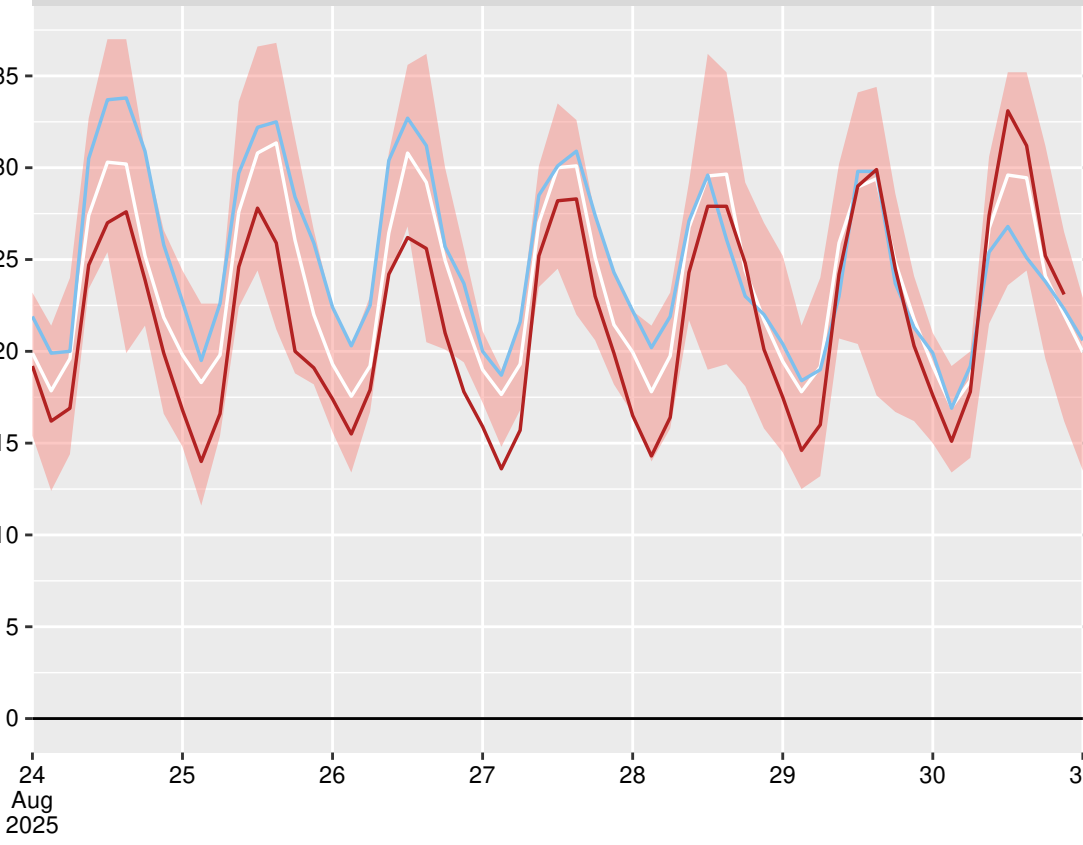
Разград (15549), 2025-08-30 21:00:00
