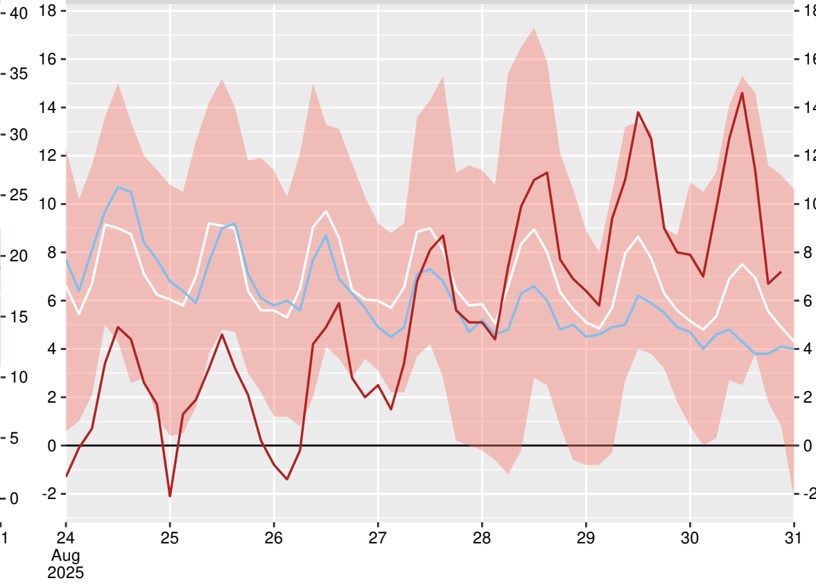
Ловеч (15525), 2025-08-30 21:00:00
