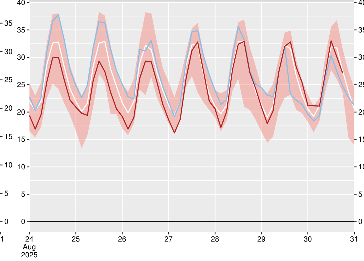
София (15614), 2025-08-30 21:00:00
