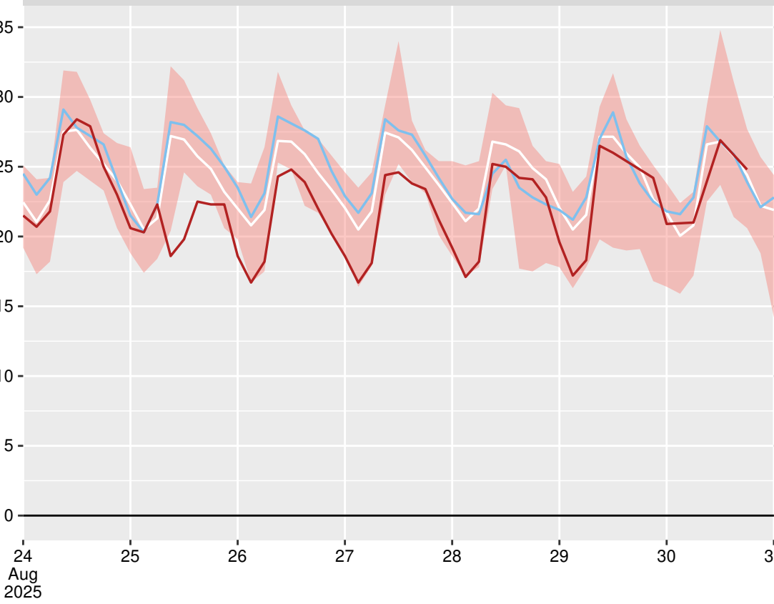
Видин (15502), 2025-08-30 21:00:00
