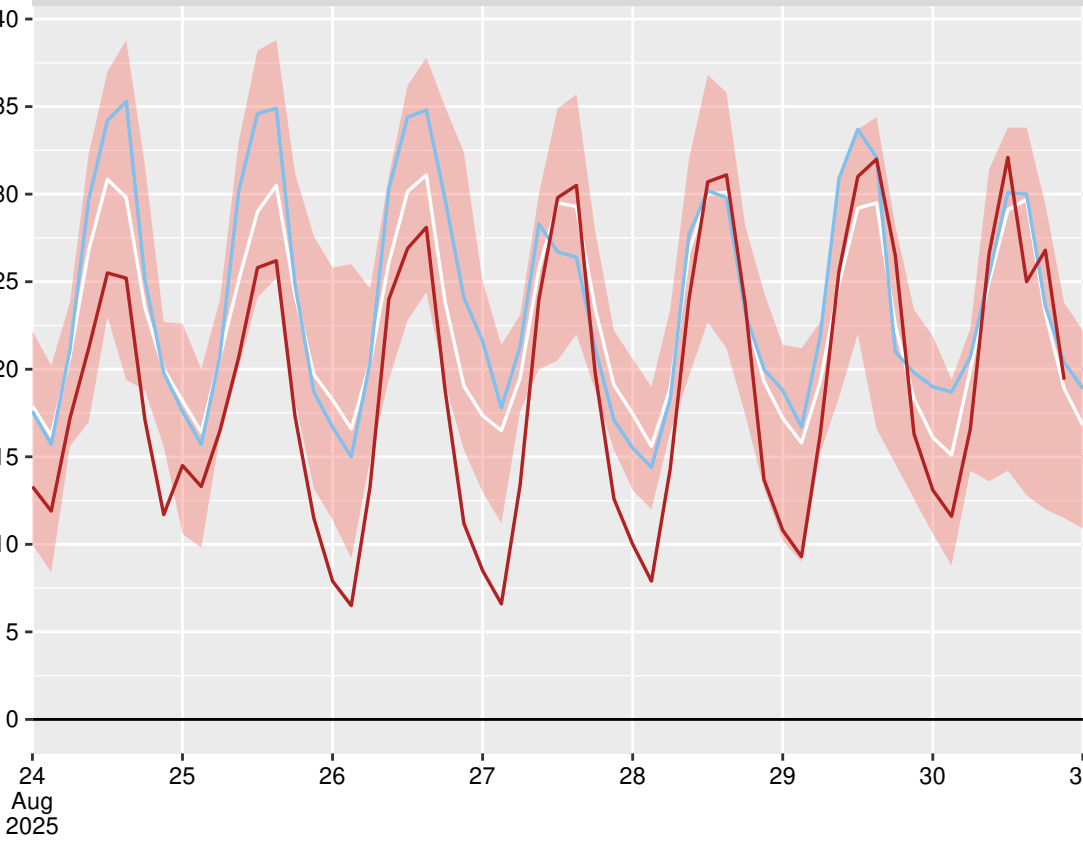
Кърджали (15730), 2025-08-30 21:00:00
