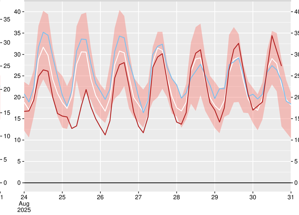
Сандански (15712), 2025-08-30 21:00:00
