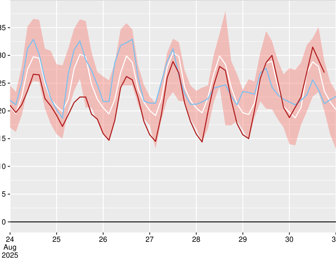
Сливен (15640), 2025-08-30 21:00:00
