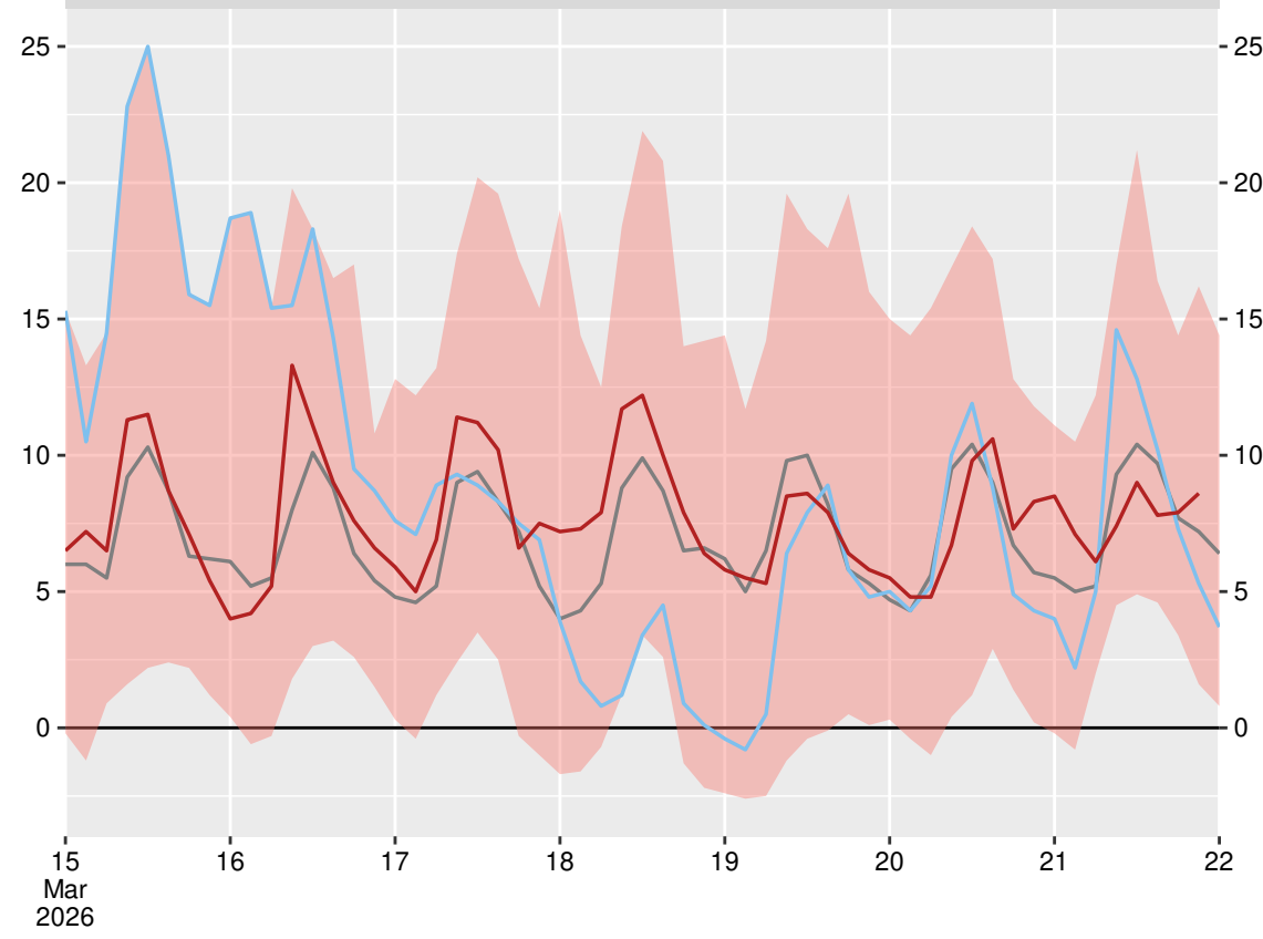
вр. Мусала (15615), 2026-03-21 21:00:00
