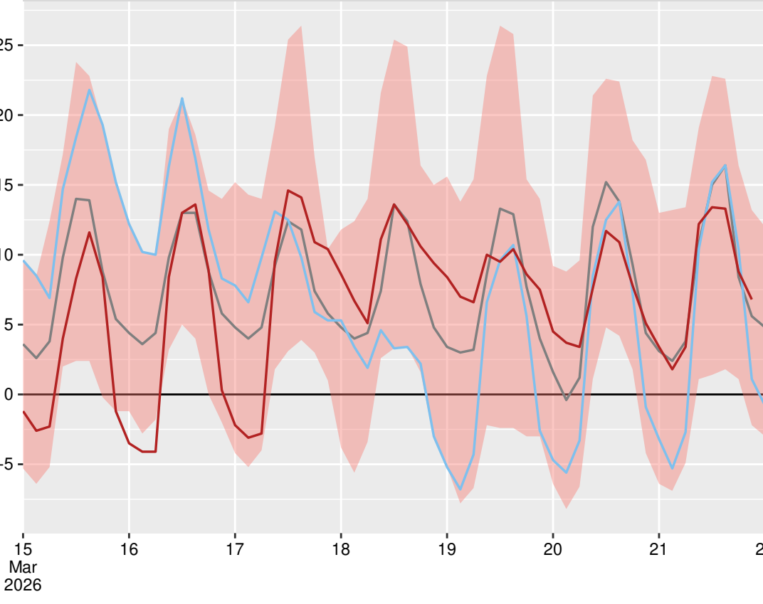
Кърджали (15730), 2026-03-21 21:00:00
