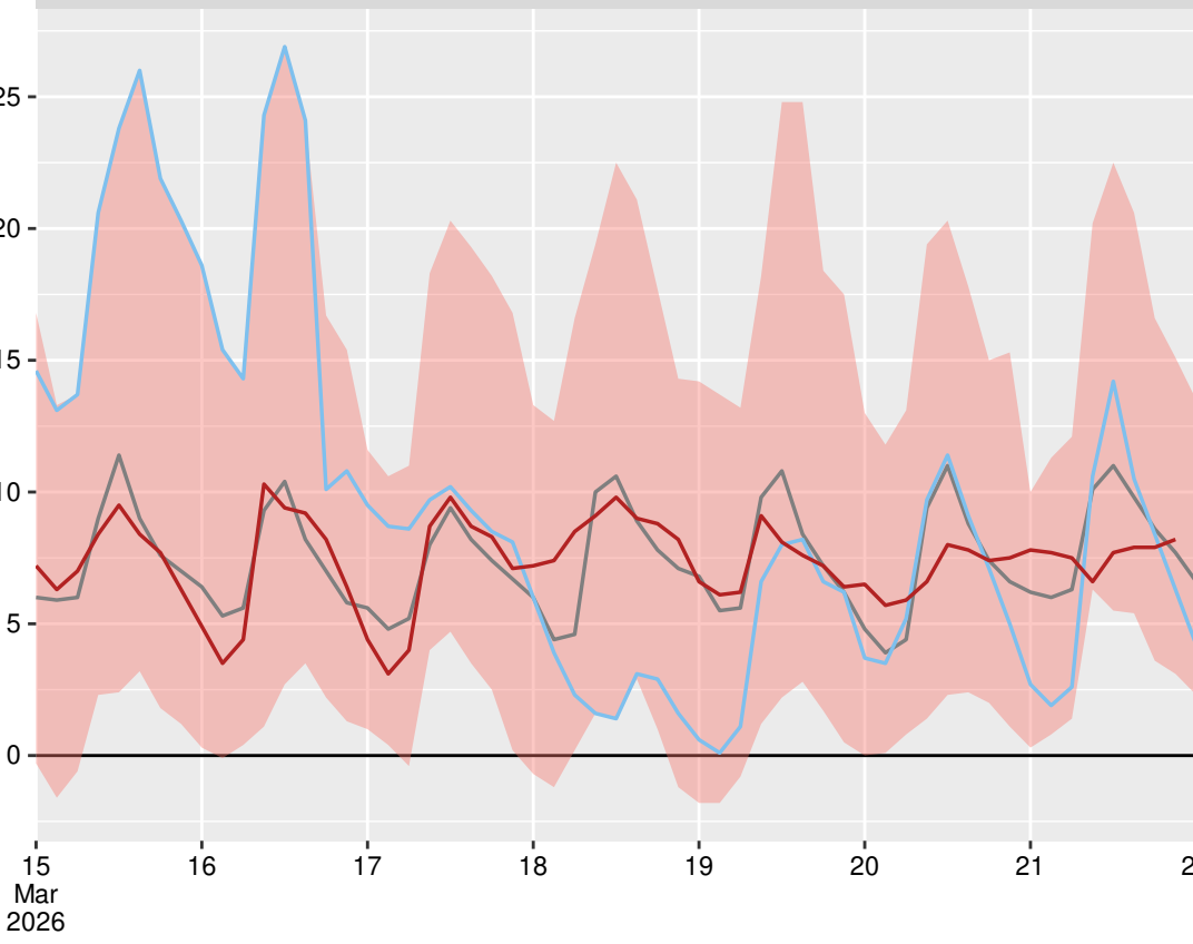
Видин (15502), 2026-03-21 21:00:00
