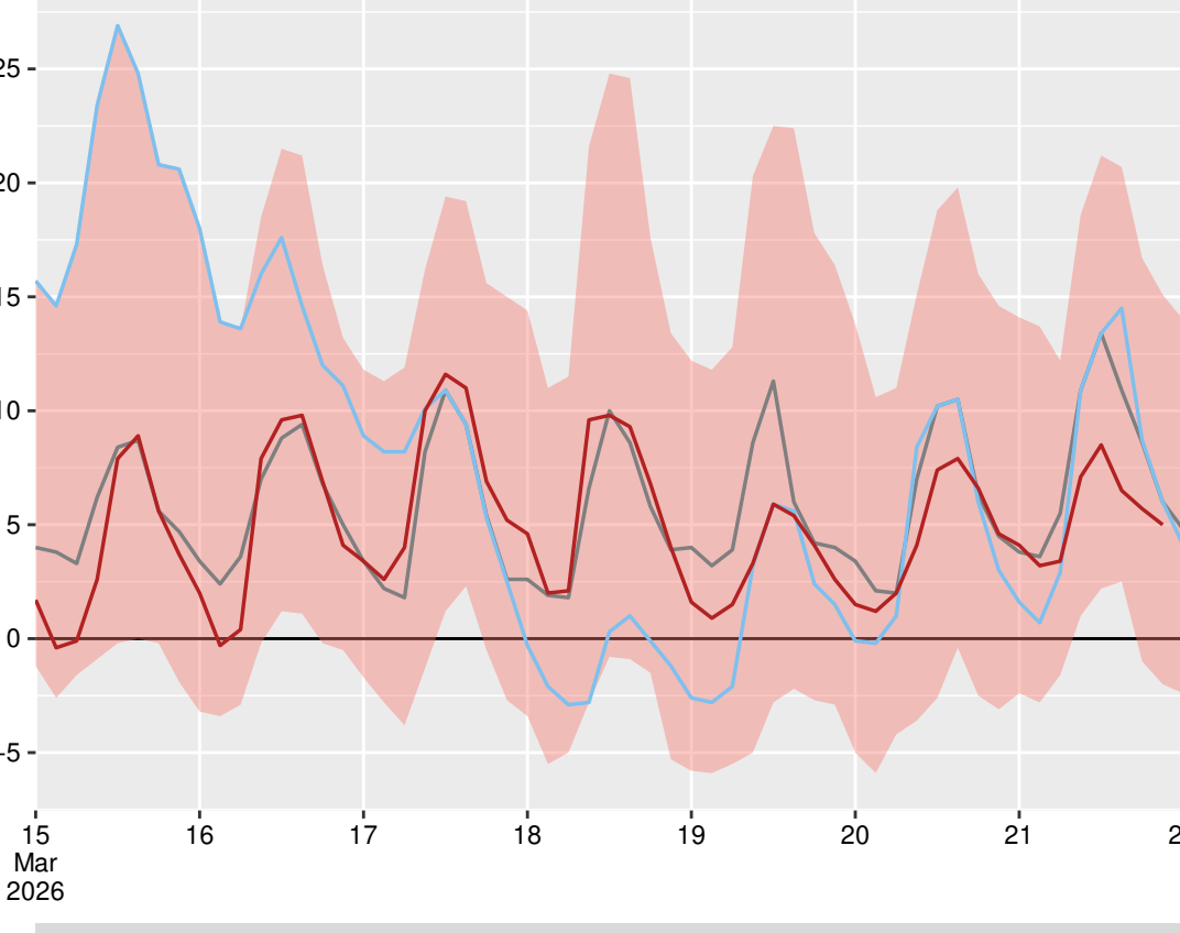
Сливен (15640), 2026-03-21 21:00:00
