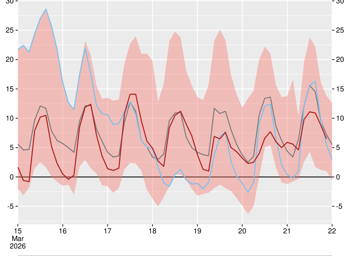
Сандански (15712), 2026-03-21 21:00:00
