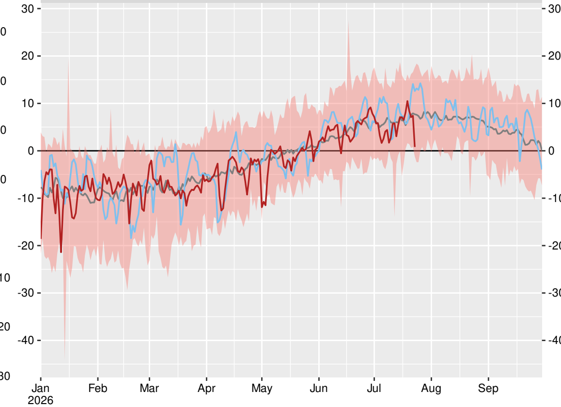
Ловеч (15525), 2026-07-23
