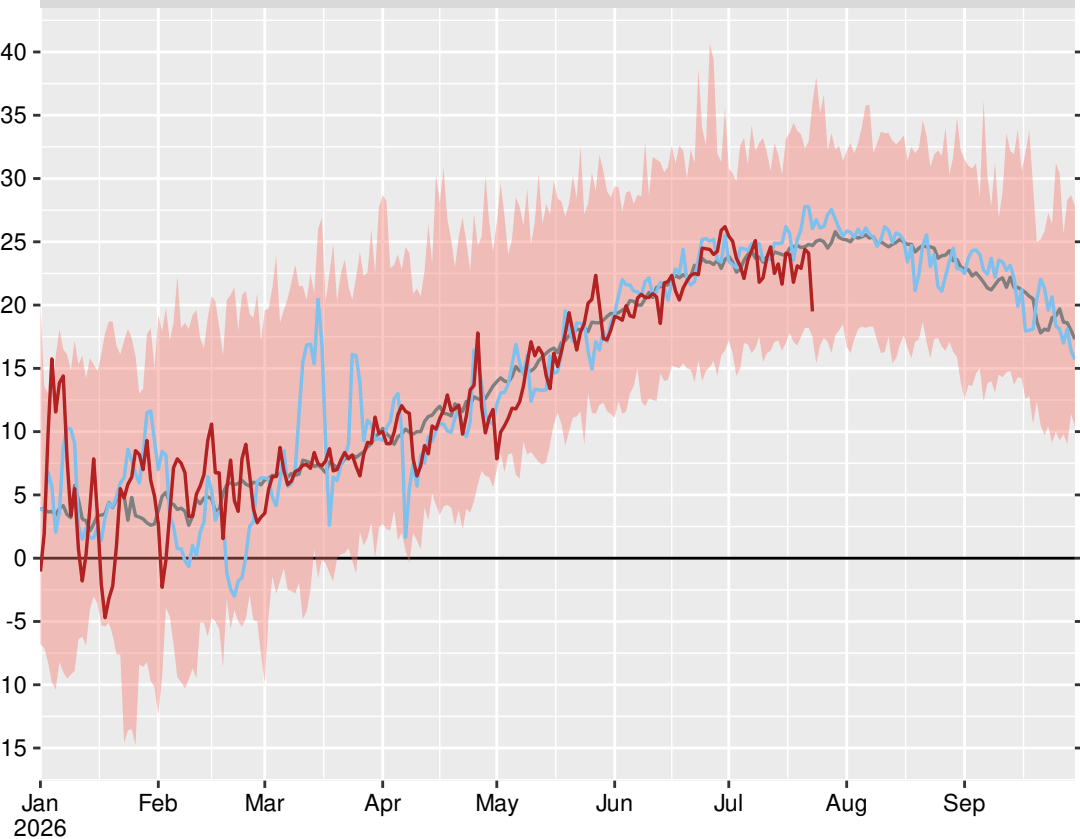
Видин (15502), 2026-07-23
