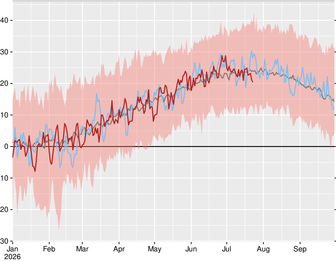
Кърджали (15730), 2026-07-23
