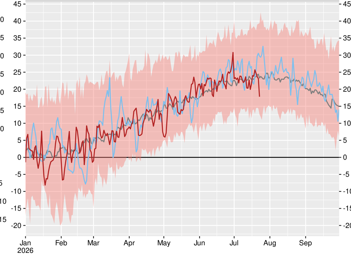
Сандански (15712), 2026-07-23
