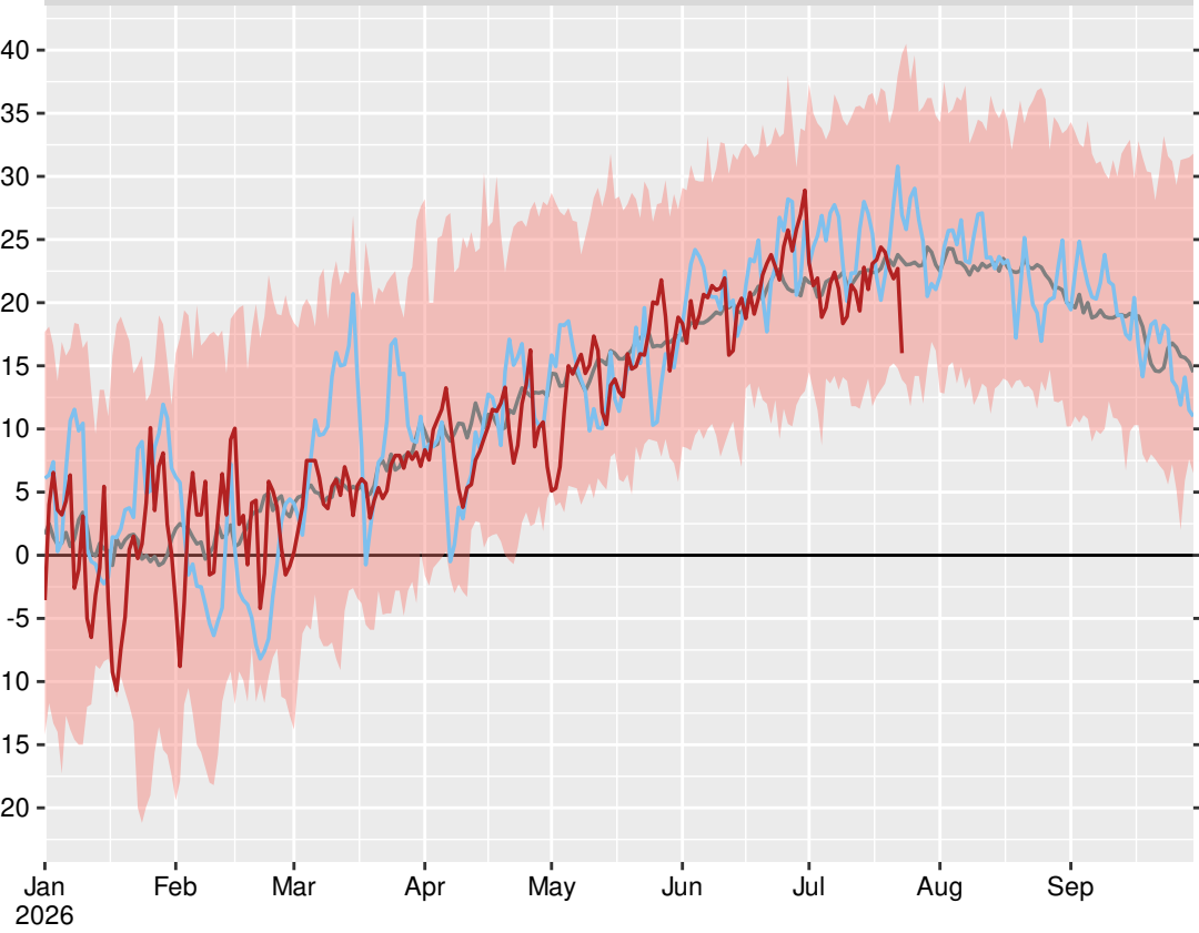
Сливен (15640), 2026-07-23
