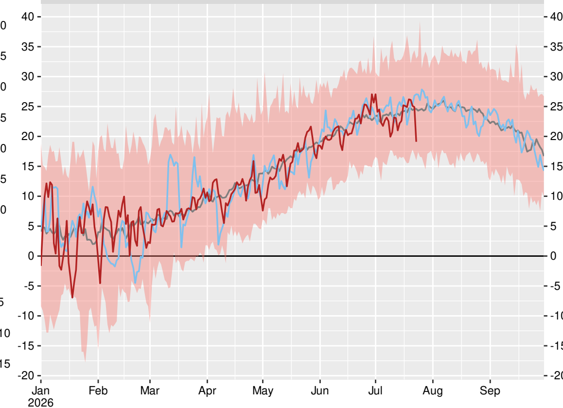
вр. Мусала (15615), 2026-07-23
