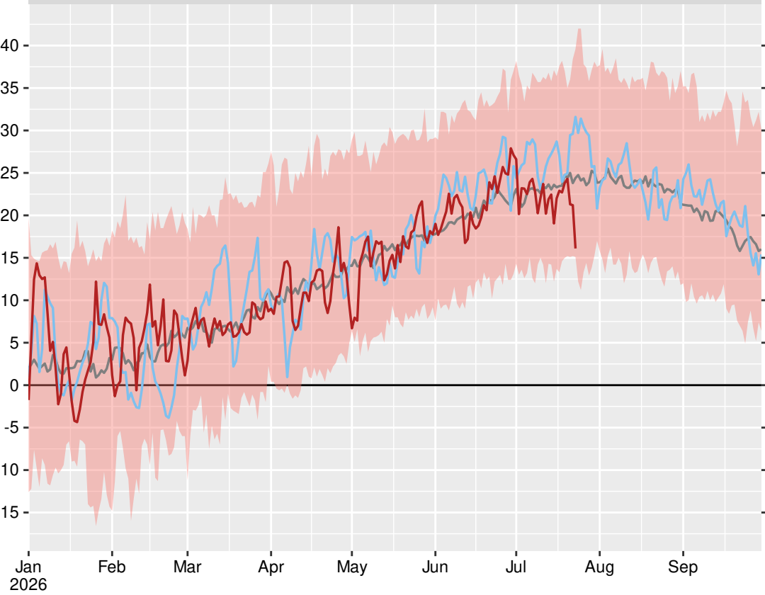
Разград (15549), 2026-07-23
