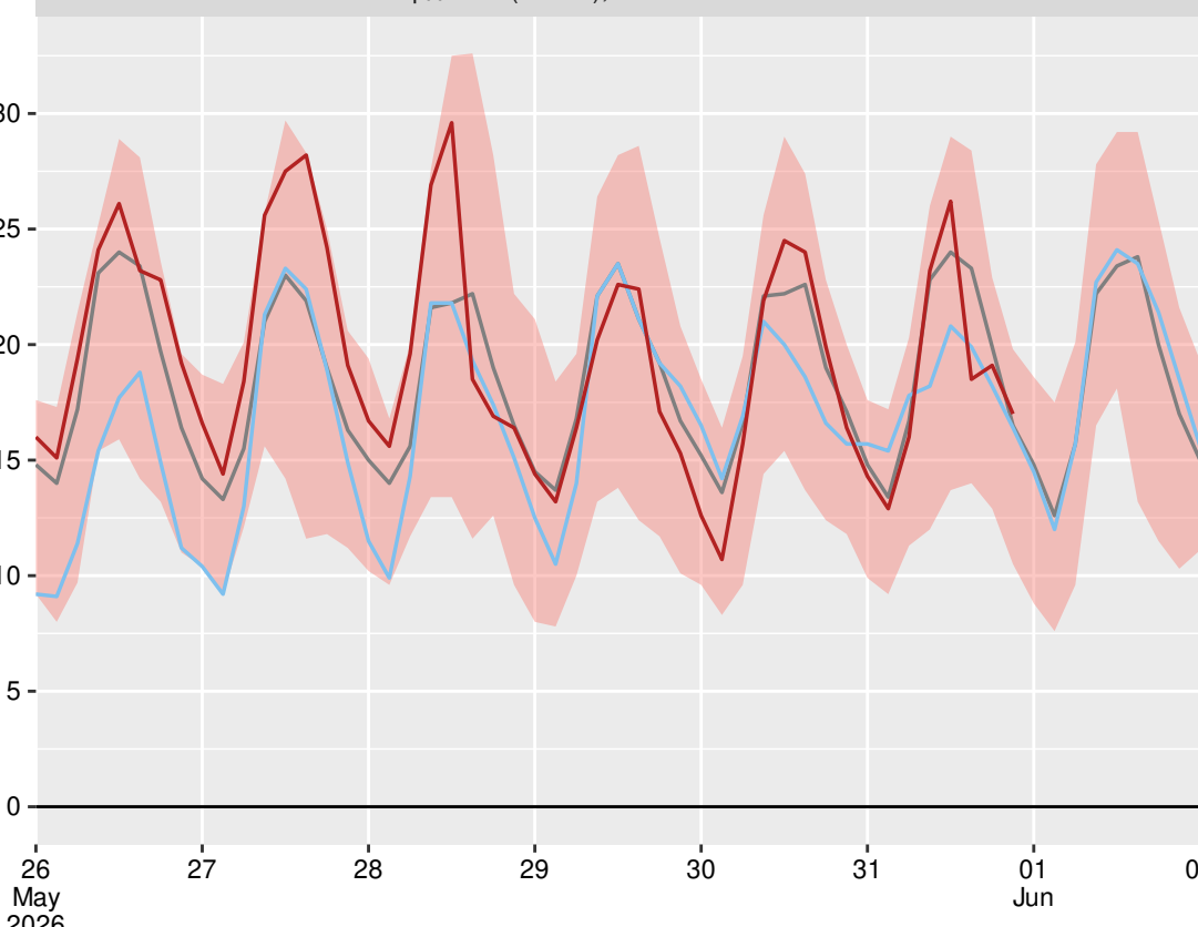
Разград (15549), 2026-05-31 21:00:00
