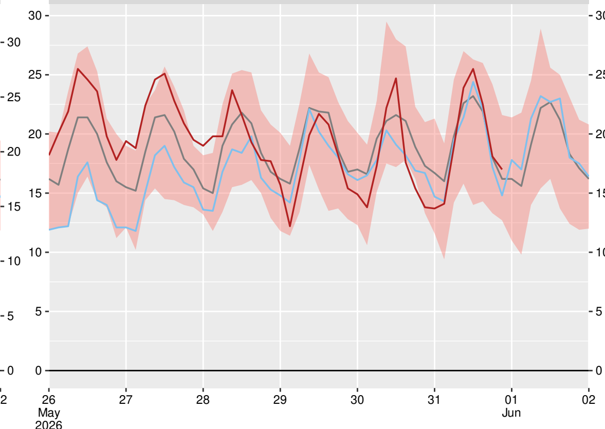
вр. Мусала (15615), 2026-05-31 21:00:00
