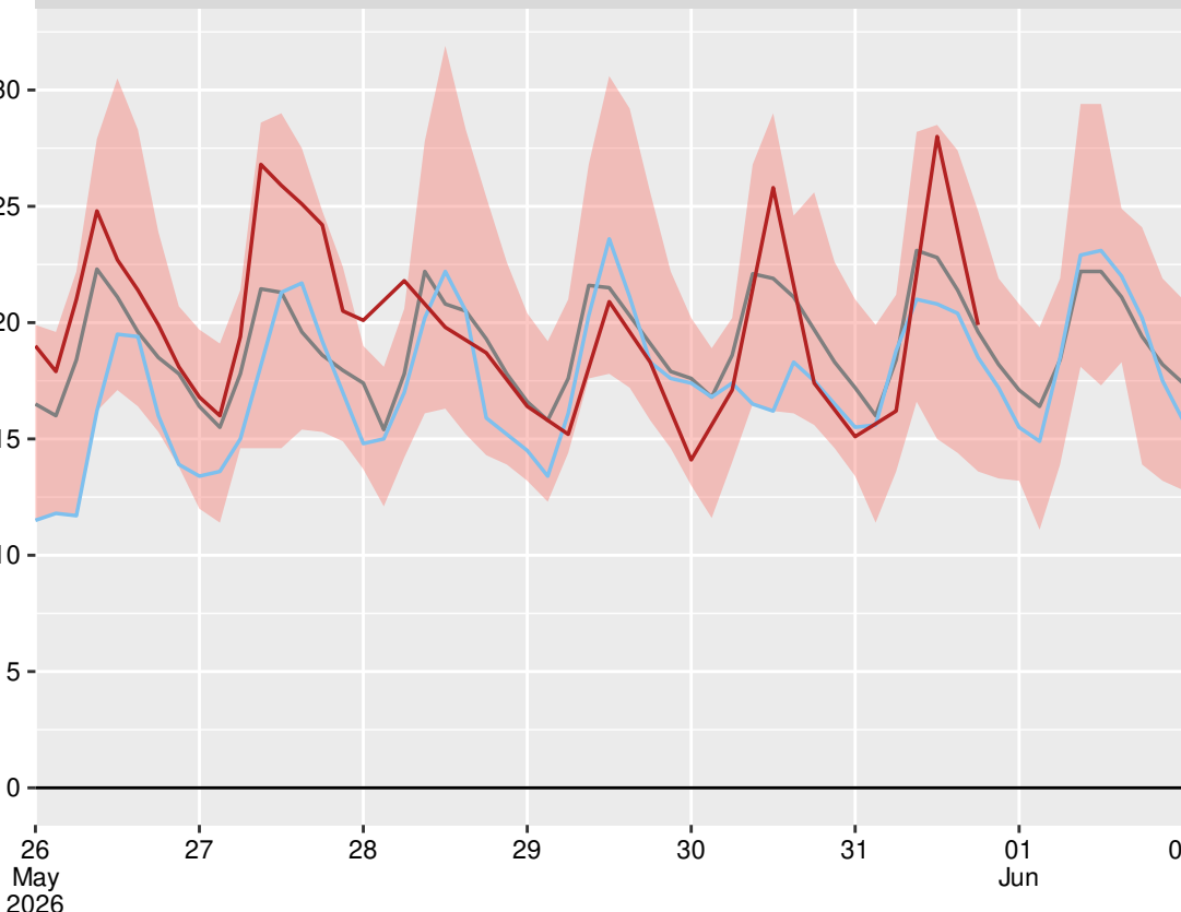
Видин (15502), 2026-05-31 21:00:00
