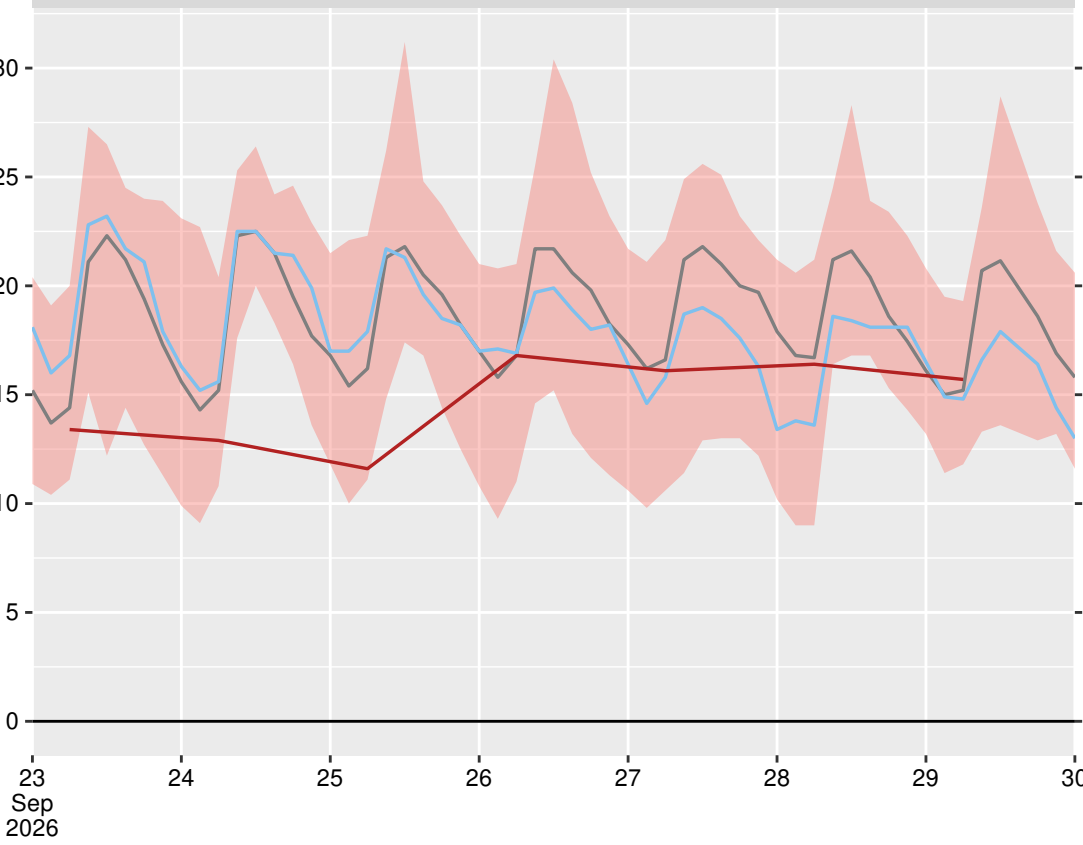
Видин (15502), 2026-09-29 06:00:00
