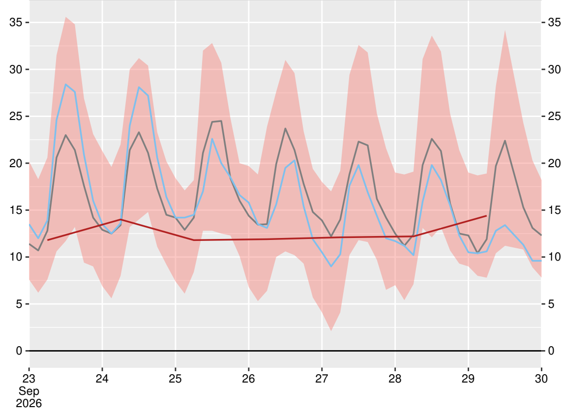
Сандански (15712), 2026-09-29 06:00:00
