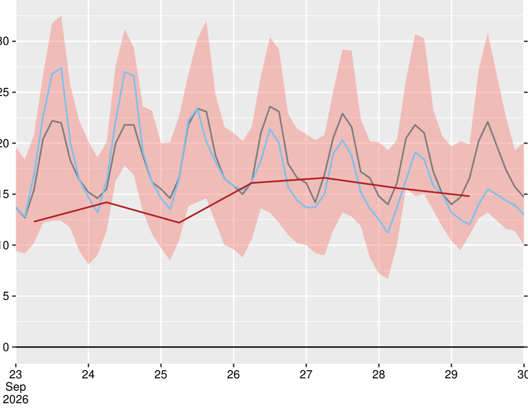
Сливен (15640), 2026-09-29 06:00:00
