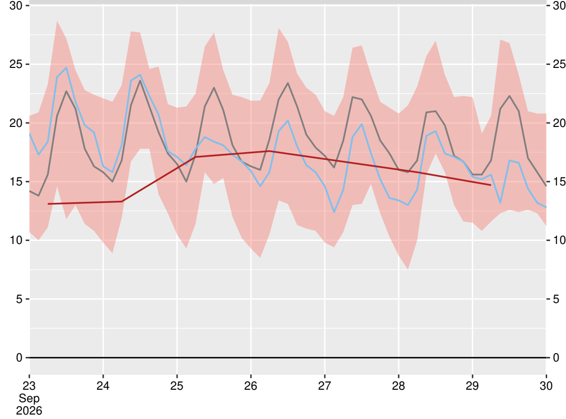
вр. Мусала (15615), 2026-09-29 06:00:00
