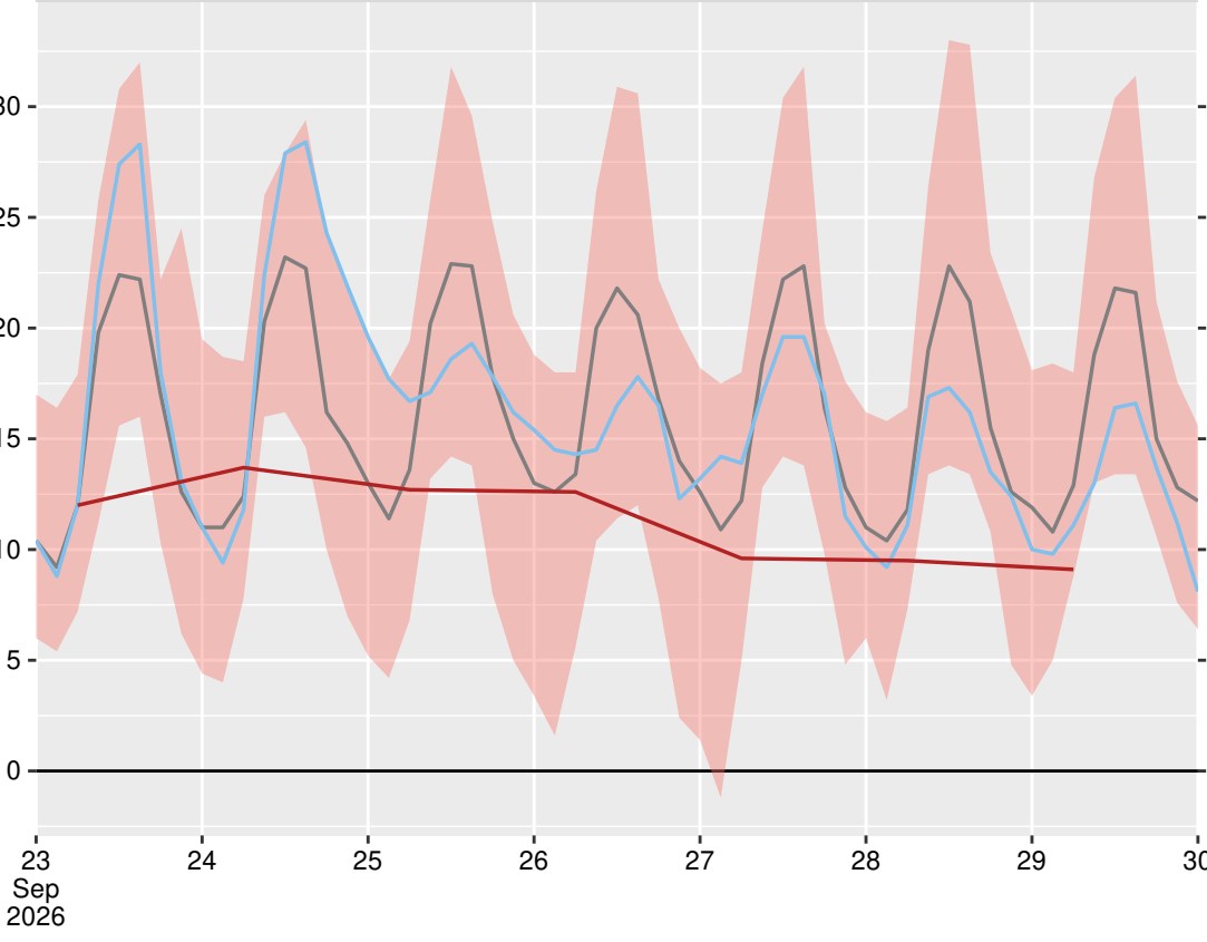
Кърджали (15730), 2026-09-29 06:00:00
