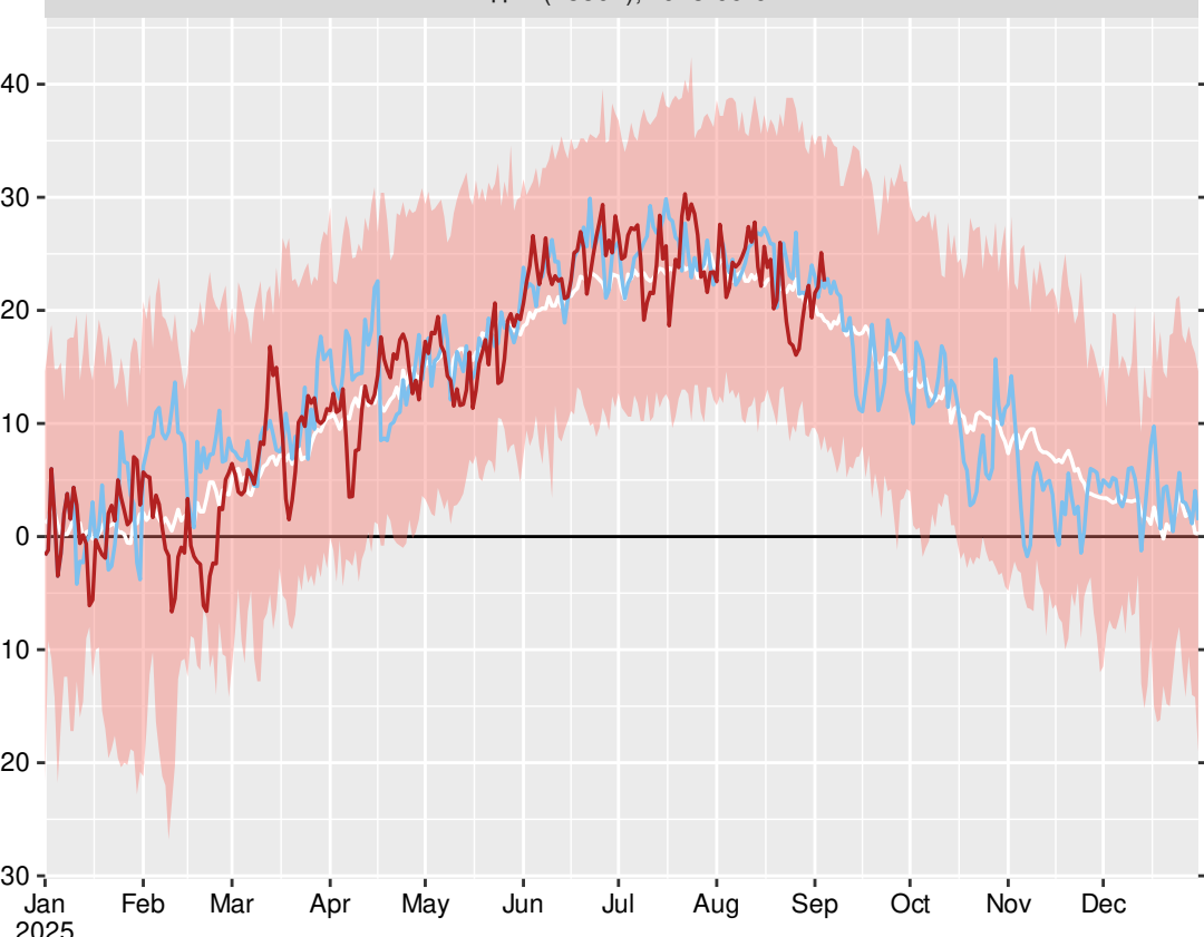
Кърджали (15730), 2025-09-04
