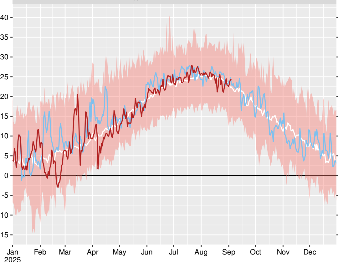
Видин (15502), 2025-09-04
