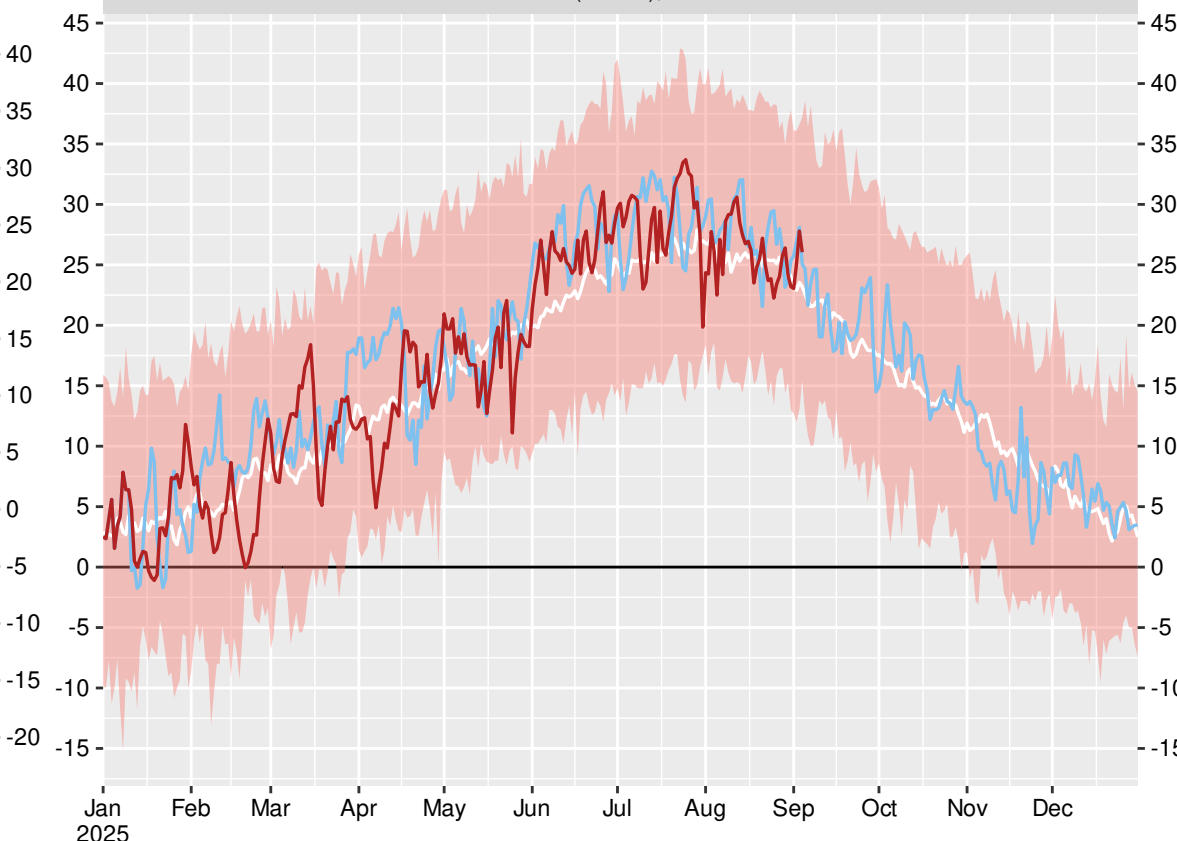
София (15614), 2025-09-04
