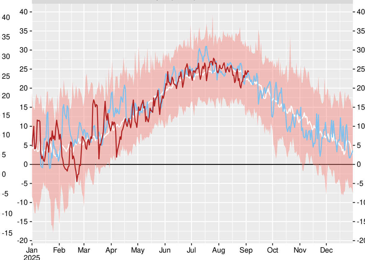
вр. Мусала (15615), 2025-09-04
