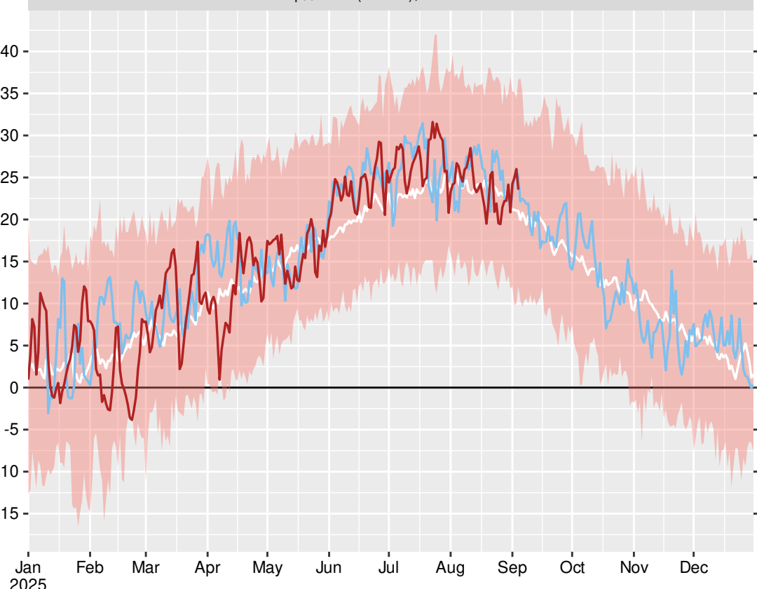
Разград (15549), 2025-09-04
