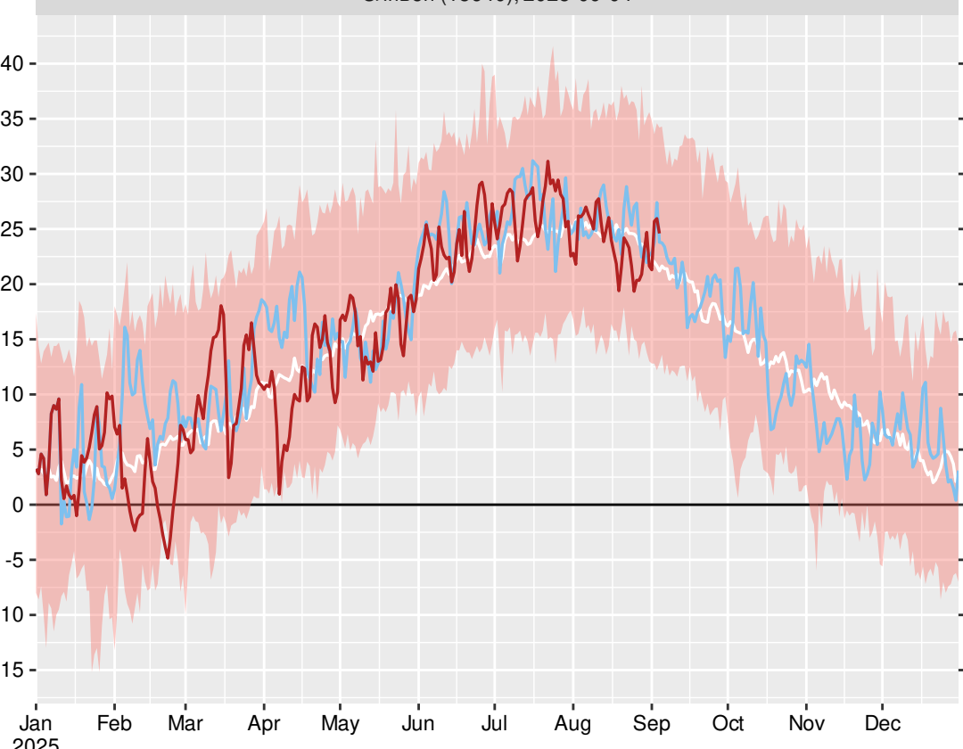
Сливен (15640), 2025-09-04
