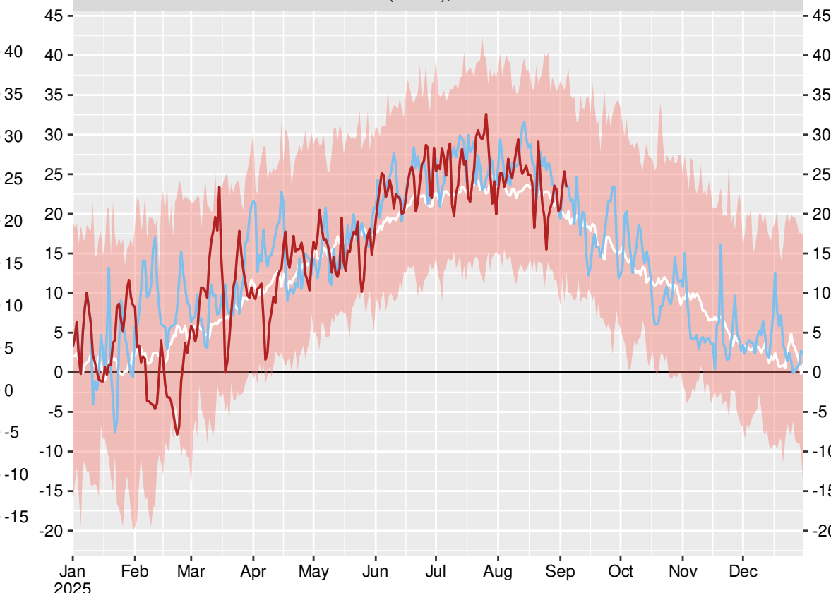
Сандански (15712), 2025-09-04
