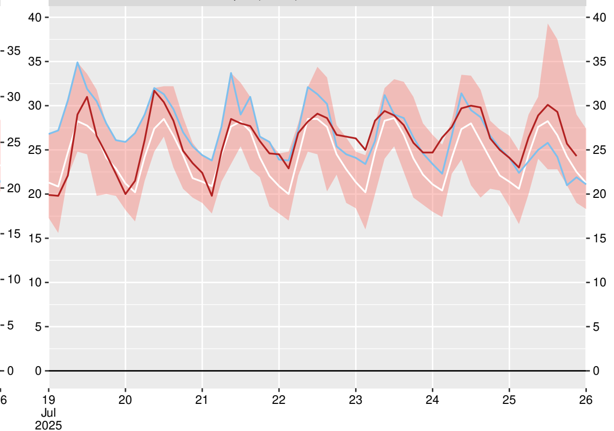
вр. Мусала (15615), 2025-07-25 21:00:00
