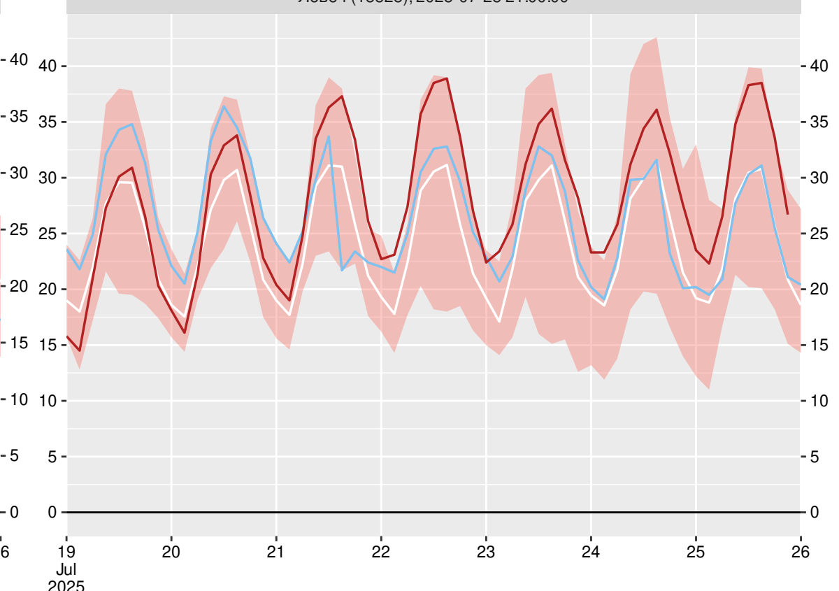
Сандански (15712), 2025-07-25 21:00:00
