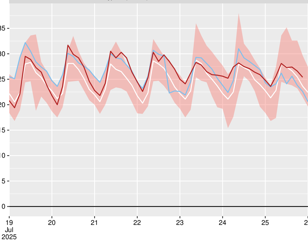
Видин (15502), 2025-07-25 21:00:00
