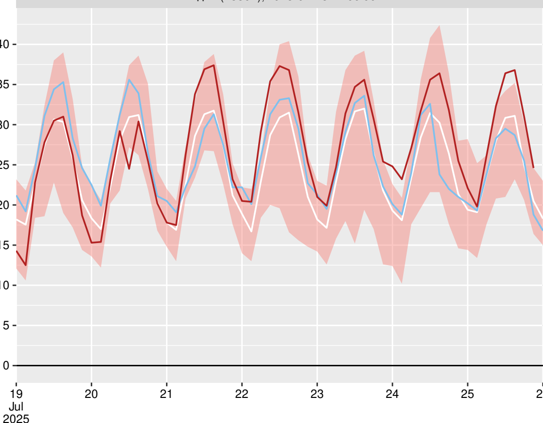
Кърджали (15730), 2025-07-25 21:00:00
