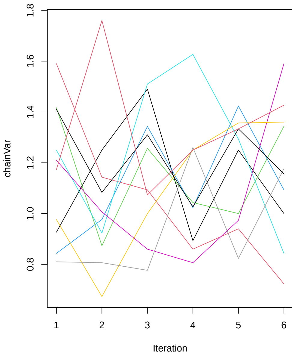
sat12 chainVar
