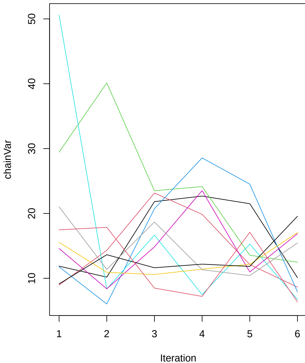
finc12 chainVar
