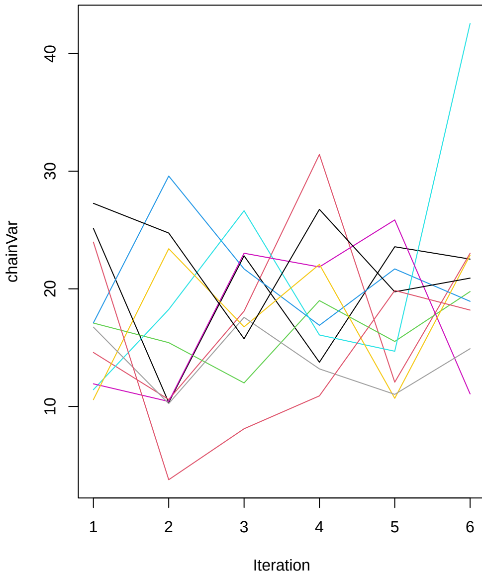
cdar12 chainVar
