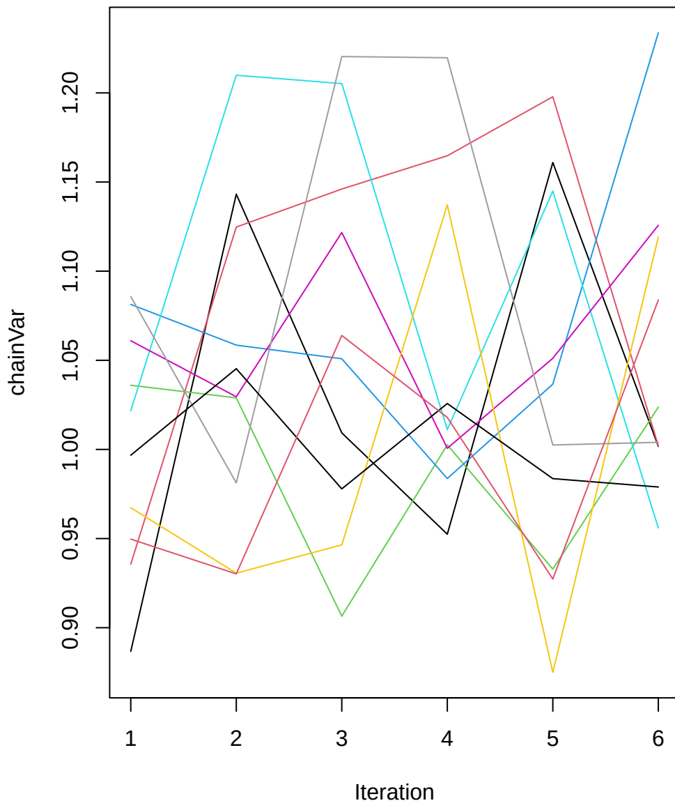
pinc12 chainVar
