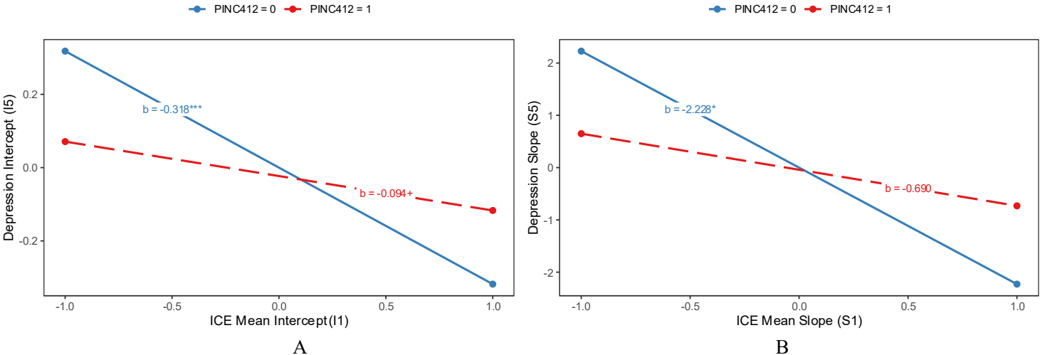
【历史计分 / 插补版本：仅供追溯，不用于当前假设判定】图 4.5.4: PP-LGCM moderation effects of closeness traj on depressive traj。注：PINC412=0/1 分别表示无个人收入/有个人收入；共同基线设为 0，保留组别主效应，纵轴为条件预测的相对水平。+ p<.10, * p<.05, ** p<.01, *** p<.001。
