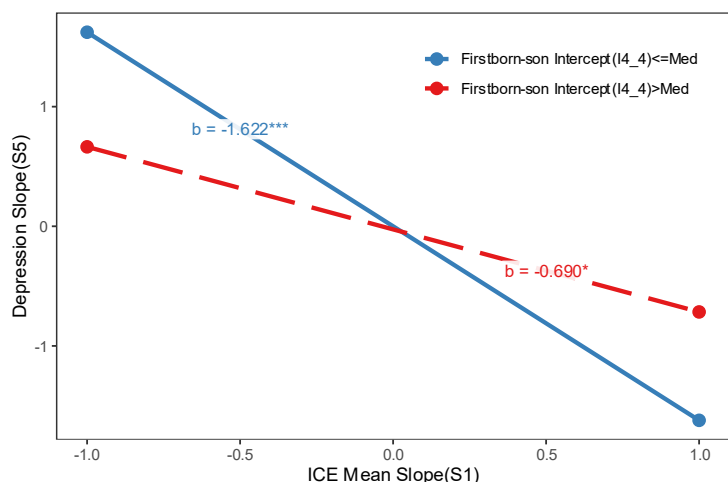
【历史计分 / 插补版本：仅供追溯，不用于当前假设判定】 Figure 4.4.2.4: PP-LGCM Sib_diff4_4 moderation effects of closeness mean traj on depressive traj_MI_TICs_r。注：调节变量按中位数分为 0 ( \leq 中位数) 和 1 ( > 中位数)；共同基线设为 0，保留调节变量主效应，曲线表示条件预测的相对水平。组间斜率差异须依据交互项检验，不能由各组显著性不同直接判断。
