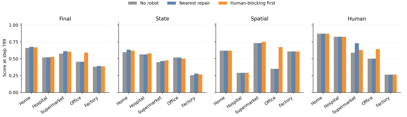
图 2. 800 step fixed schedule 规则调度基线对比。柱状图比较 no-robot、nearest-repair 和 human-blocking-first 在五个 base scenes 上的综合分、状态分、空间分和人类事件分。
