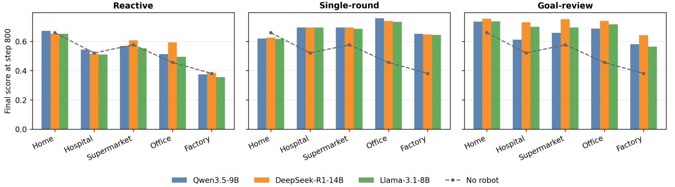
图 3. 800 step 模型主干对比实验。柱状图为 reactive、single-round 和 goal-review 三种机器人策略在 Qwen3.5-9B、DeepSeek-R1-14B 和 Llama-3.1-8B 上的最终综合分，灰色虚线为对应场景的无机器人基线。
