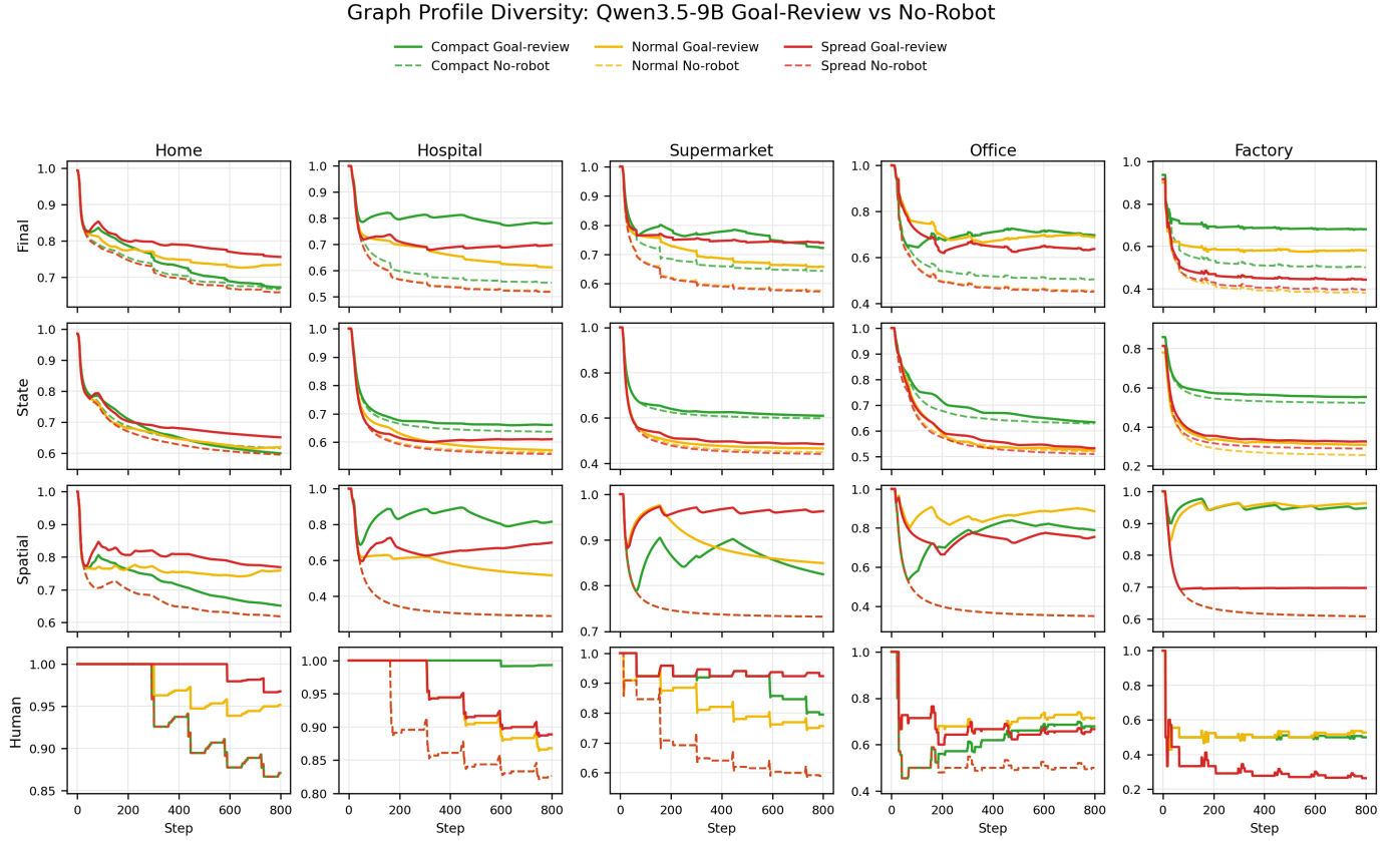
图 4. Graph 多样性实验。实线为 Qwen3.5-9B goal-review, 虚线为对应 no-robot raw baseline; 颜色表示 compact、normal 和 spread 三种 profile。各子图为累计平均 final/state/spatial/human 分数。
