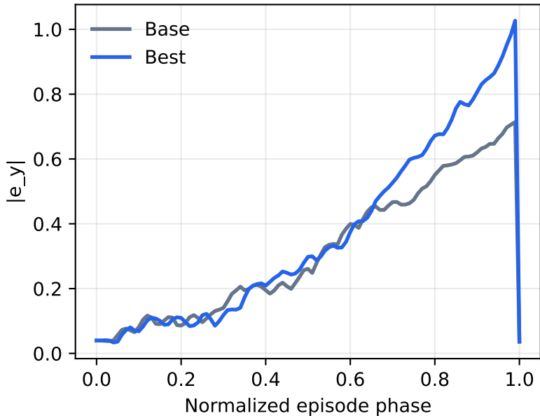
Centerline error
