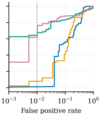
AD-Shift
