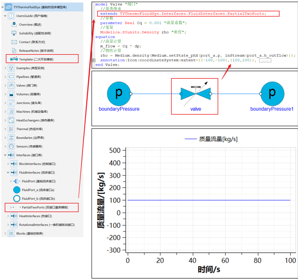
图 4-1 自定义阀门模型开发
