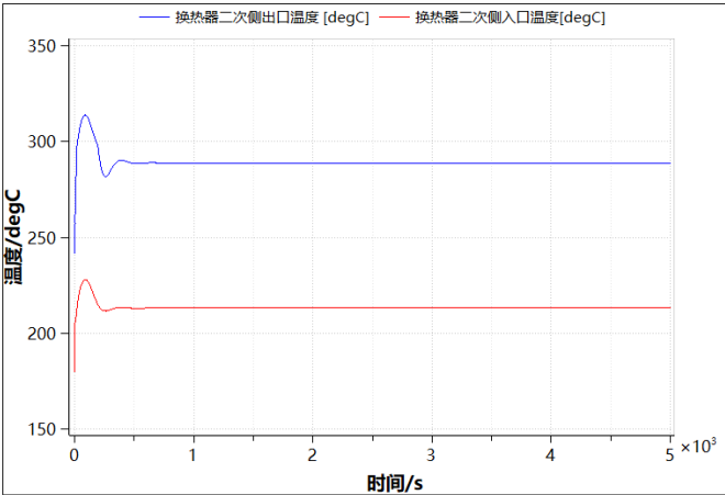
图 5-12 换热器出入口温度曲线
