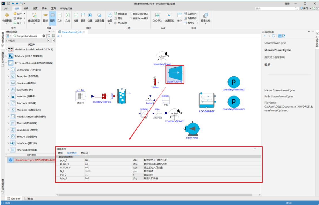
图 3-6 集中参数级汽轮机参数设置
