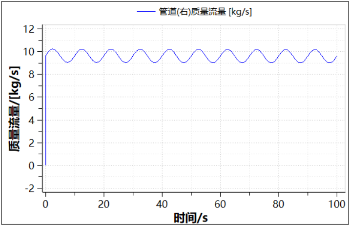
图 5-8 管道（右）质量流量计算结果
