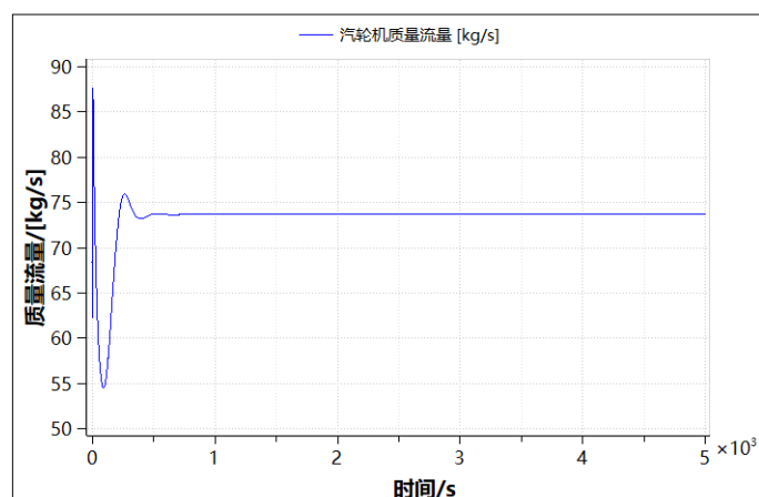
图 5-13 汽轮机质量流量曲线
