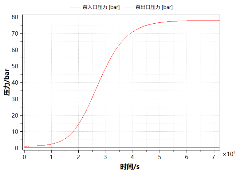
图 5-4 泵出入口压力曲线
