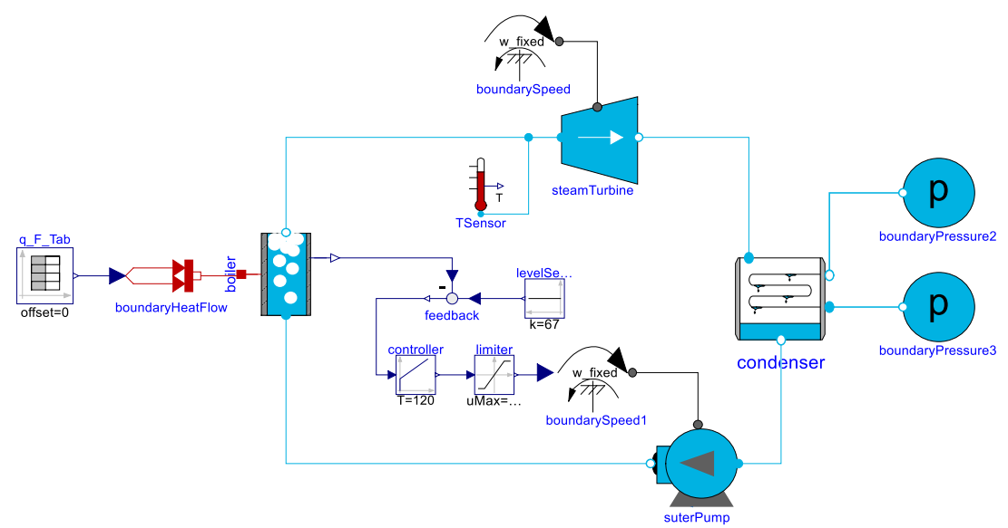
图 5-1 蒸汽动力循环系统
