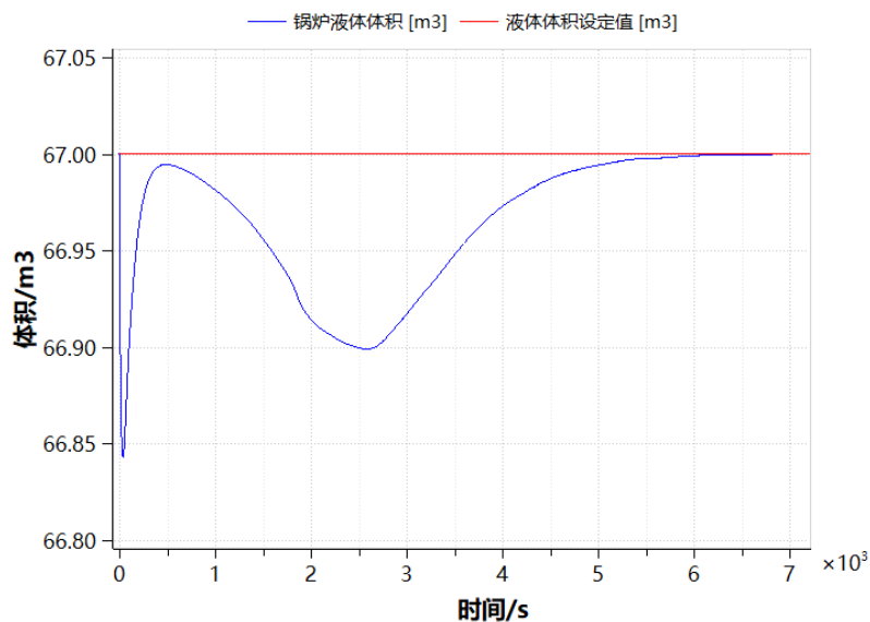
图 5-3 锅炉液体体积曲线
