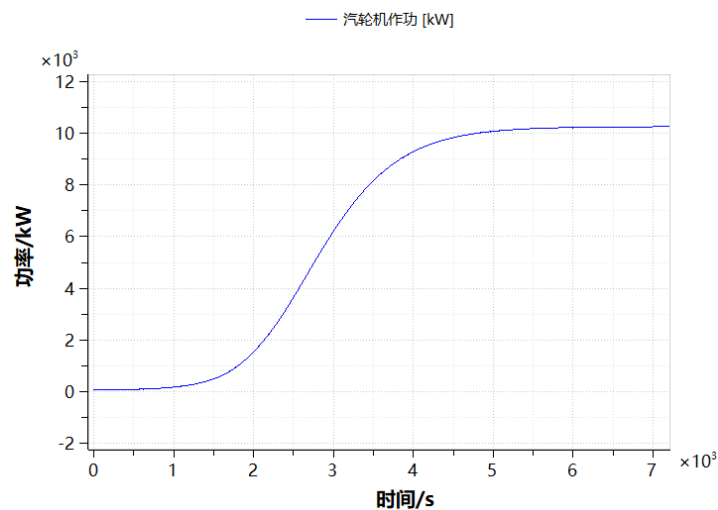
图 5-5 汽轮机做功曲线
