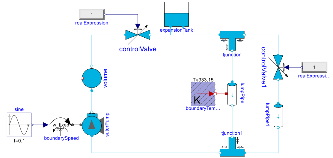
图 5-7 水箱系统
