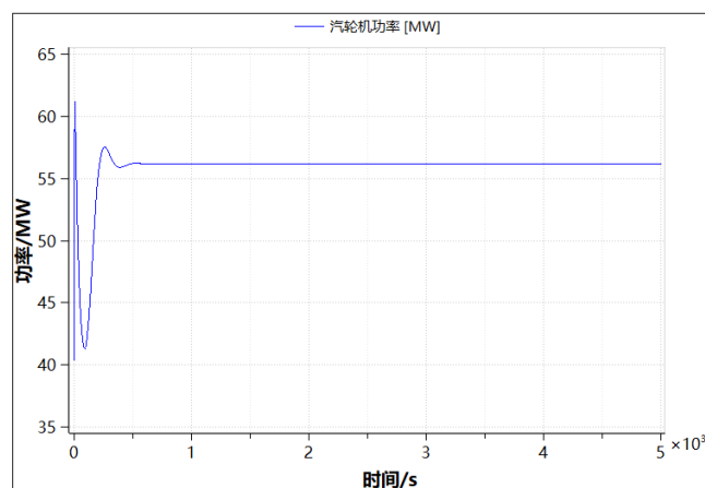
图 5-14 汽轮机功率曲线
