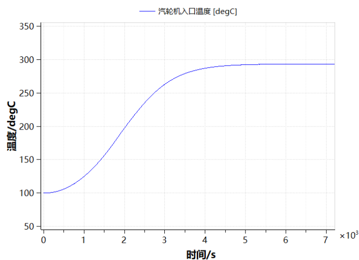
图 5-6 汽轮机入口温度曲线
