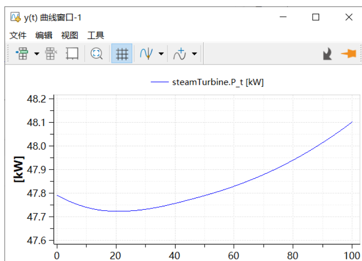
图 3-8 汽轮机做功曲线
