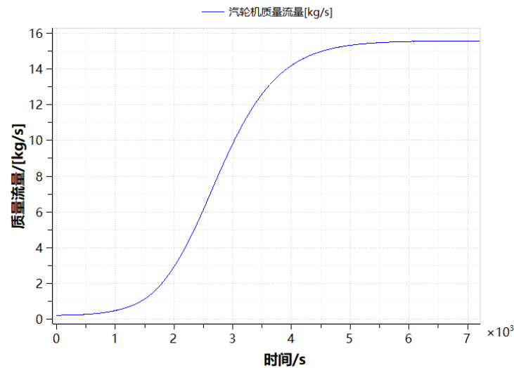
图 5-2 汽轮机质量流量曲线
