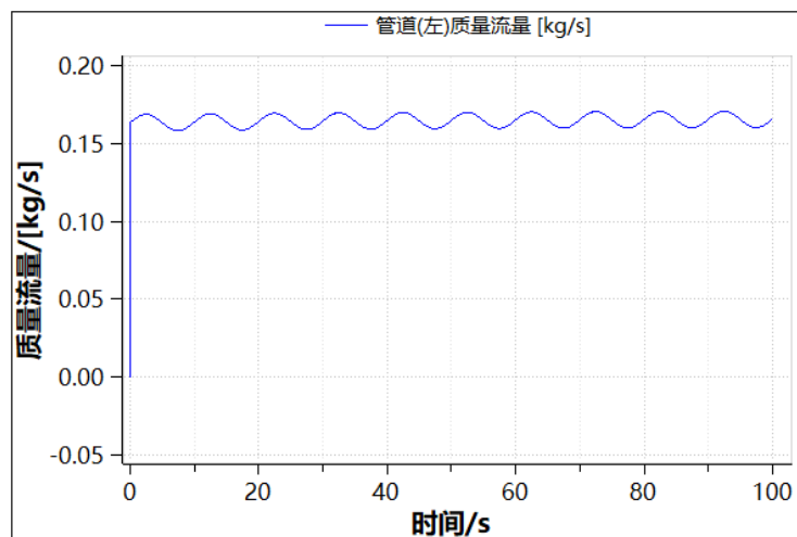
图 5-9 管道（左）质量流量计算结果
