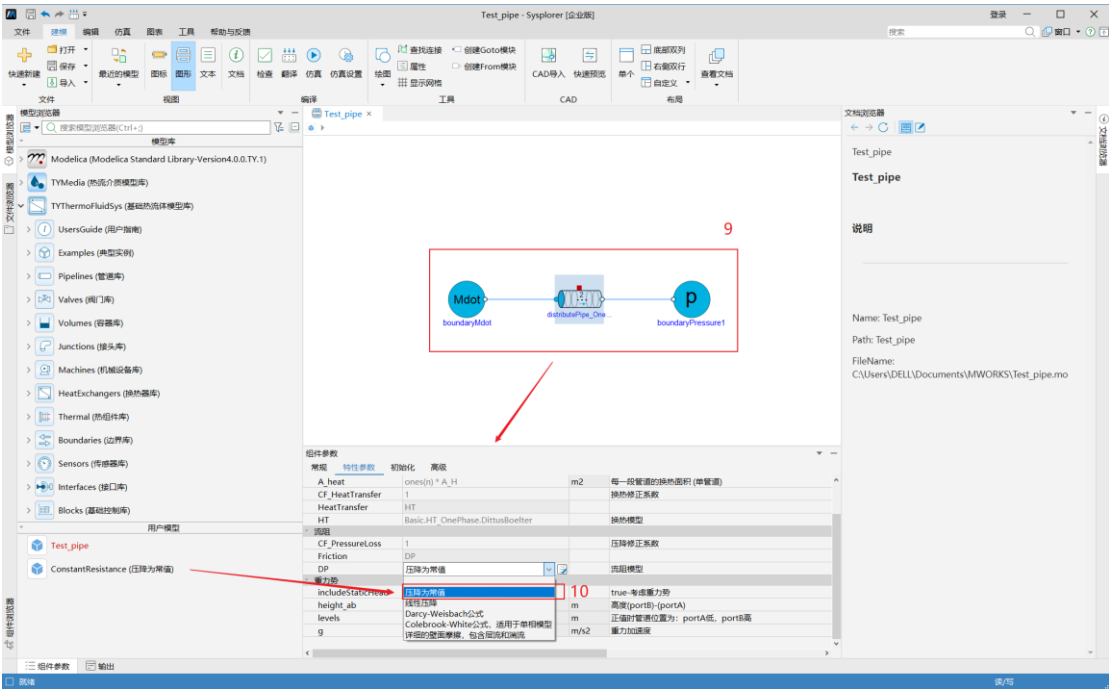
图 4-27 接口连线搭建系统模型以及参数设置
