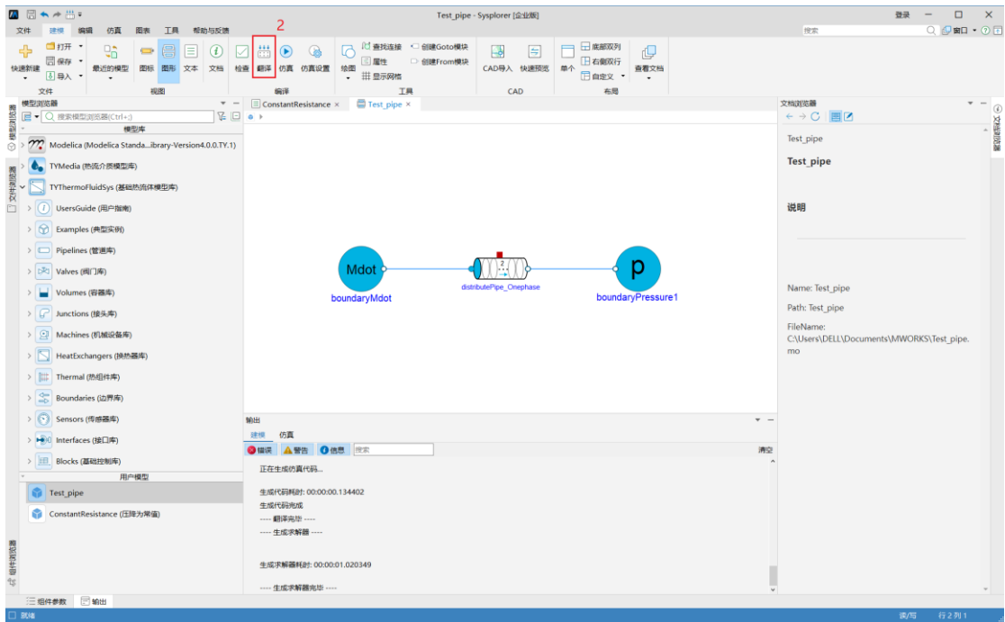
图 4-29 管道测试系统模型编译结果
