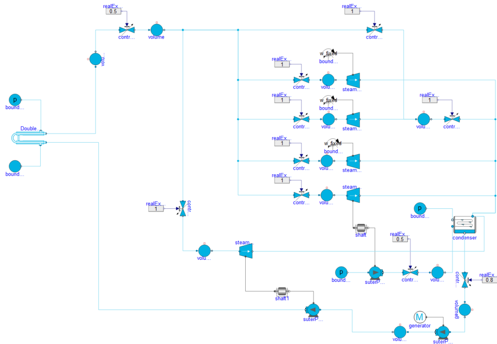
图 5-11 二回路系统
