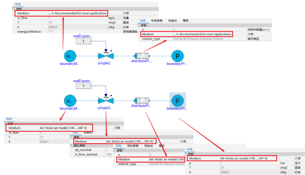
图 6-1 介质传递说明
