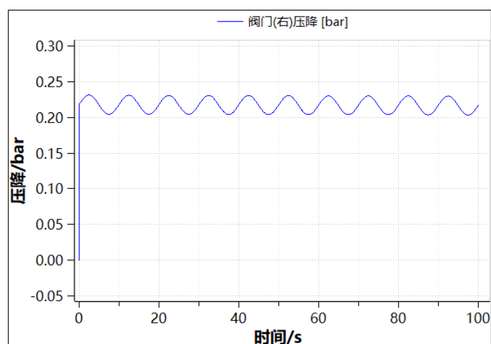
图 5-10 阀门（右）压降计算结果
