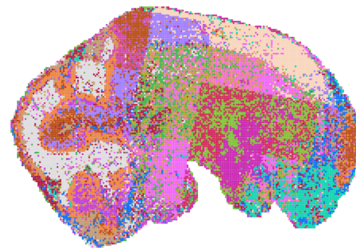
SToFM
