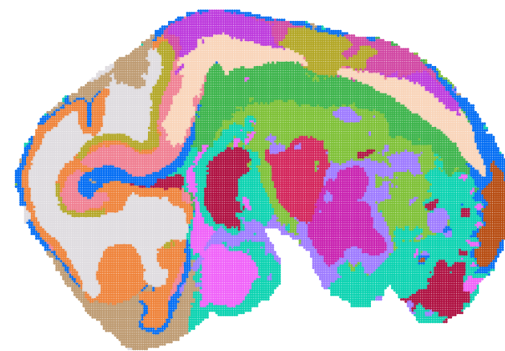
STAGATE
