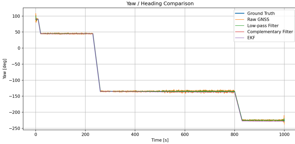
Şekil 8. Yaw / yönelim karşılaştırması.
