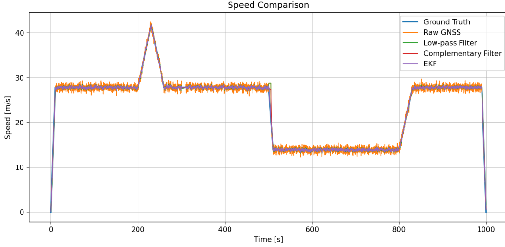
Şekil 7. Hız profili karşılaştırması (100 km/sa \approx 27.8 m/s, 150 km/sa \approx 41.7 m/s).
