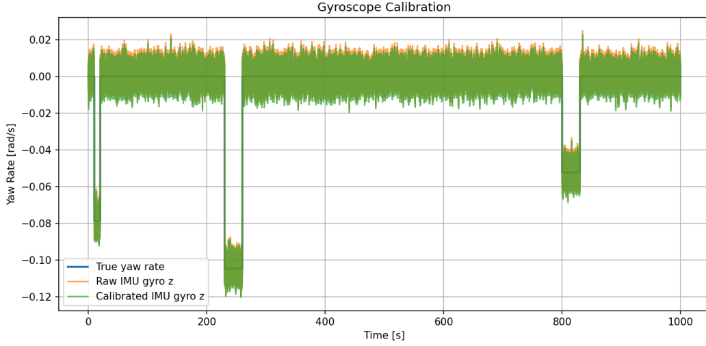
Şekil 4. Jiroskop: gerçek yaw-rate, ham ve kalibre edilmiş ölçüm.
