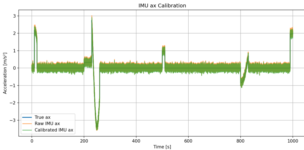
Şekil 3. IMU x eksen ivmesi: gerçek, ham ve kalibre edilmiş.
