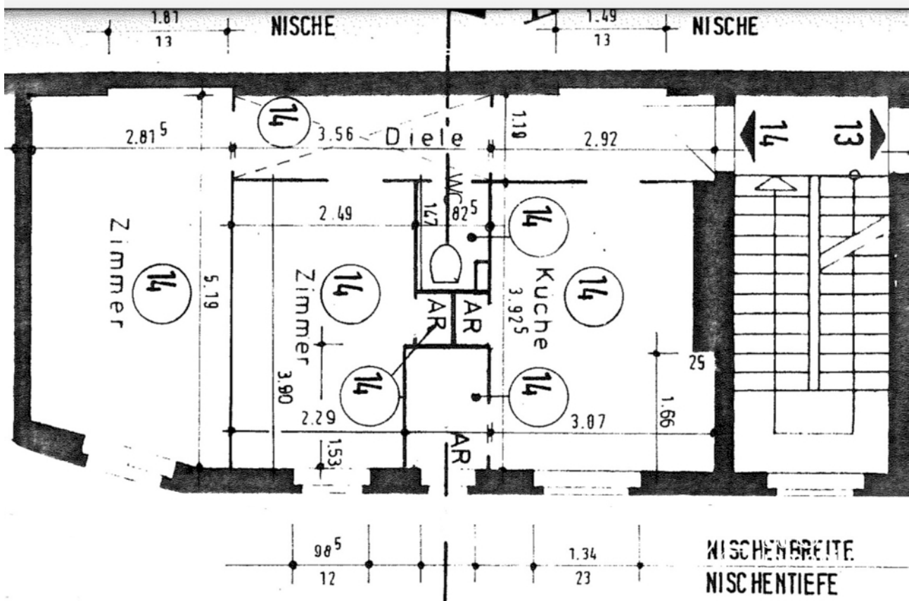
Grundriss 1909
