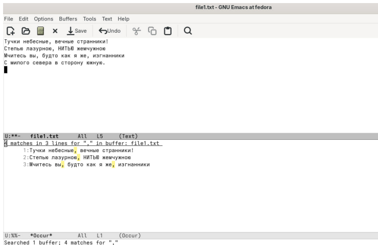
Рисунок 15: подтверждение
