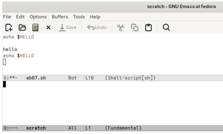
Рисунок 9: буфер scratch
