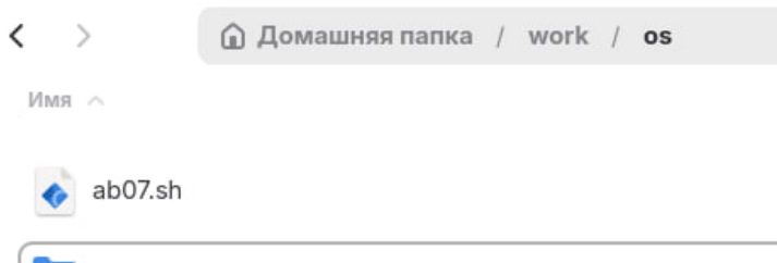
Рисунок 3: новый файл
