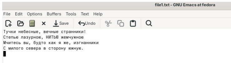
Рисунок 14: Отредактированная строка
