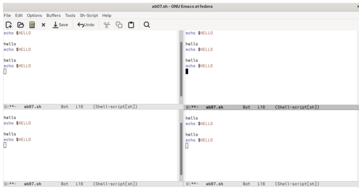
Рисунок 11: 4 новых буфера
