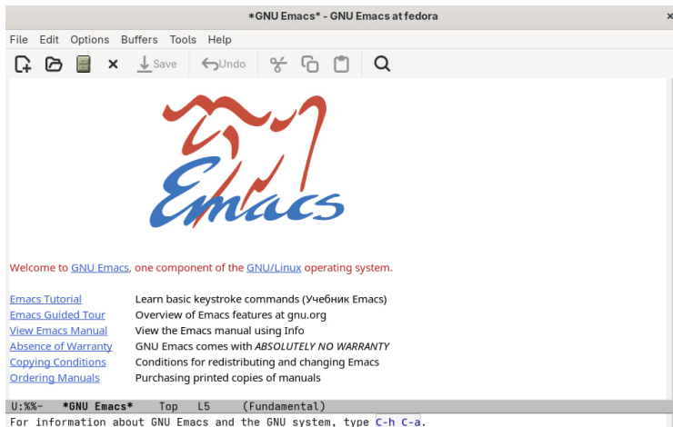
Рисунок 1: окноеmacs
