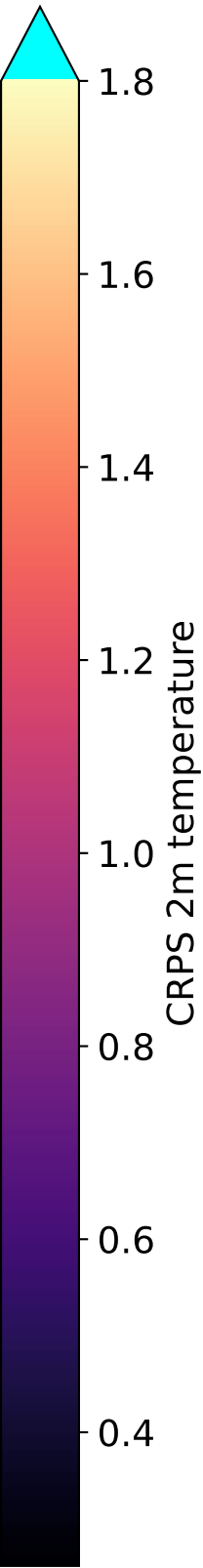
IND_UNET
