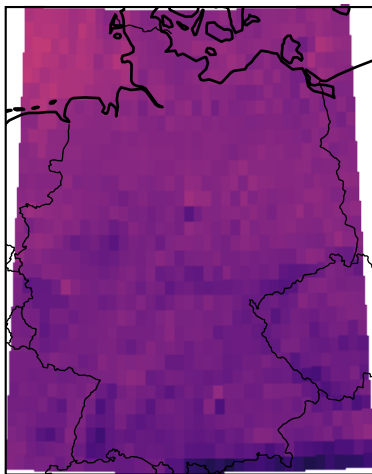
LNGM (ES)
