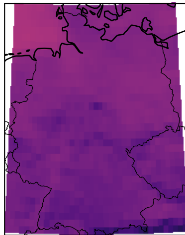
FM (UVIT)
