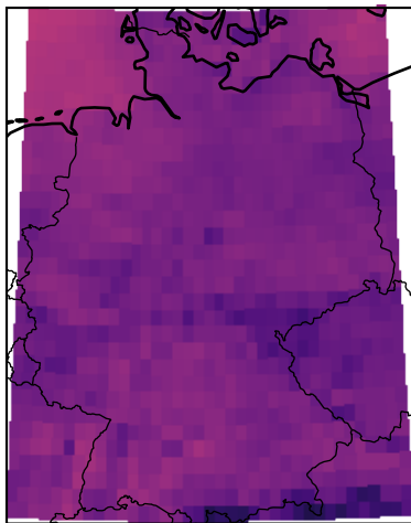
EMOS
