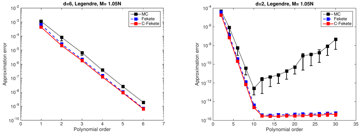
图 11 扩散方程 d = 2 与 d = 6 的 QoI 逼近误差 ( u(0.5, y) , 随机系数为类 KL 展开的余弦级数)。CFP 与 AFP 的曲线几乎重合, 都显著低于随机采样。确定性点集在超定区是免调参的选择。
