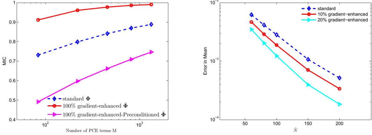
图 16 左: MIC 随 gPC 项数的变化 ( d = 3 , n = 80 ): 预条件后的 梯度增强矩阵在全部项数上保持最低常数, 验证预条件的尺度无关性。右: 随机椭圆 PDE ( d = 10 ) 的均值误差: 梯度由伴随方程获得, 梯度增强全面占优。
