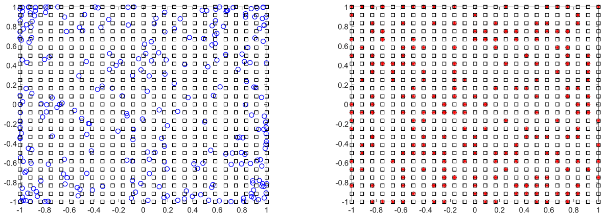
图 21 两种采样测度的散点对比（论文 2008.10121，数据为 二项 \times Poisson 模拟）。左：CSA 采样（平衡测度的经验版），点撒满了 Chebyshev 网格，大量点落在数据支撑之外；右：induced 采样，点全部落在数据样本上，采样概率按 \kappa （多项式能量）偏置，再由 1/\kappa 权重补偿，两者配对保持估计无偏。
