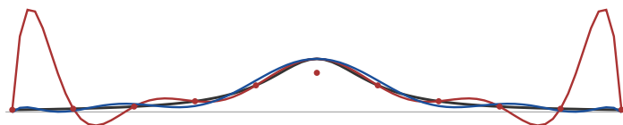
图 1 Runge 现象。两个插值多项式都精确穿过各自的 11 个节点；等距节点的插值多项式在区间两端摆出巨大的振荡（峰值约 1.9，而真函数的最大值只有 1）；Chebyshev 节点的插值全程贴住真函数。
