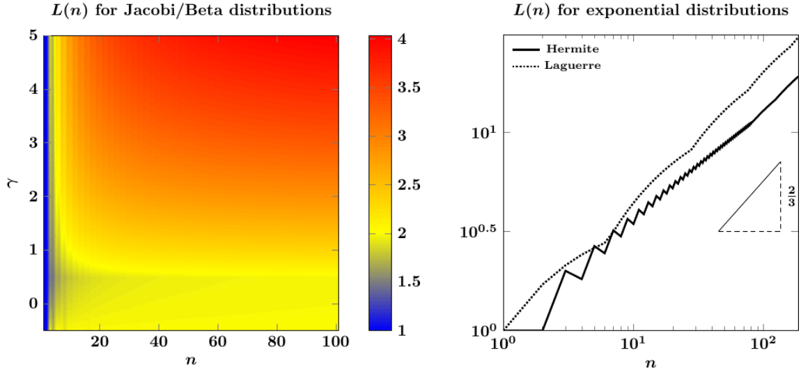
图 3 上界 L_i 的形状 (论文 1602.00995)。左: Jacobi 情形的界随参数变化, 与 n 无关; 右: Hermite/Laguerre 情形的 n^{2/3} 界。有界分布 (Legendre/Chebyshev) 是这条路的最爱: L 是常数, 样本量只比最优多 C^d 的维数代价 (数值上接近 2^d s \log^3 s \log N )。
