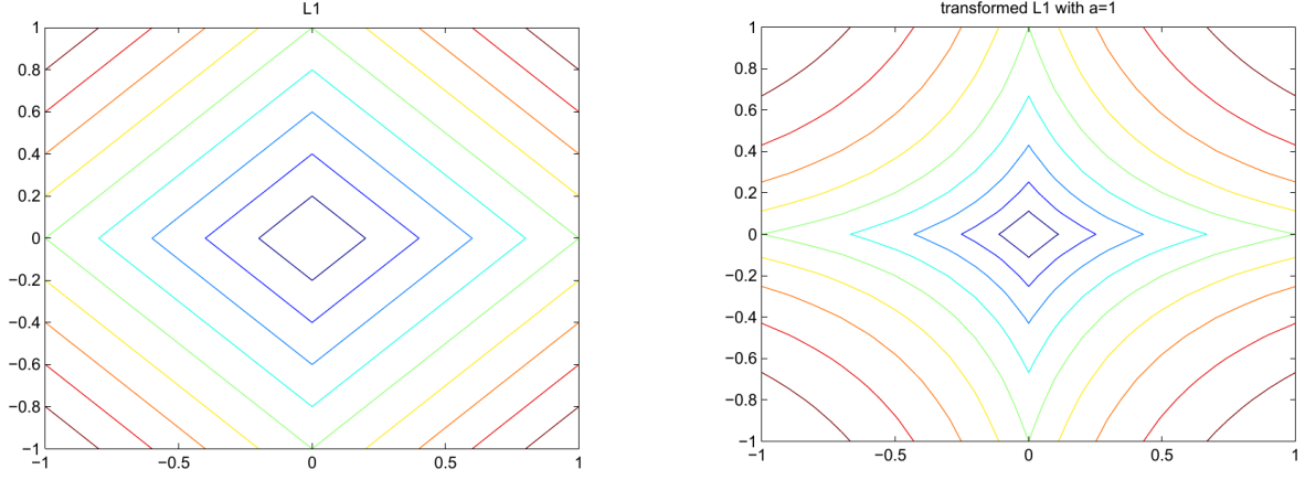
图 13 罚函数的等值线 (论文 1805.05416)。左: \ell_1 的菱形等值线; 右: TL1 ( a=1 ) 的等值线, 坐标轴附近更“尖”, 压小系数的力度更强。 a 越小等值线越贴近坐标十字 (越像 \ell_0 ), a 越大越接近左图。
