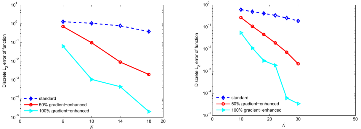
图 15 测试函数逼近误差 ( d=2 )。左: 球面函数 (梯度线性); 右: 多频正弦 (梯度振荡, 梯度增强收益最大的情形)。两图中梯度增强 (GraLeCh) 都显著低于同信息量的标准 \ell_1 。
