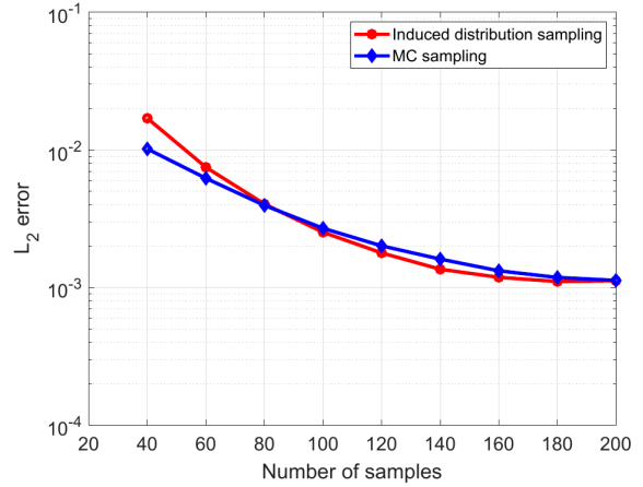
图 26 左：corner-peak 函数 (二项 \times Poisson 数据)：induced 的优势在小 M 区最明显。右：Kirchhoff 板问题的 \ell_2 误差 ( d = 10 , 3 个 KL 模态)：此时 \mu \approx \omega , induced 与 MC 相当，正是方法自己指出的适用边界。
