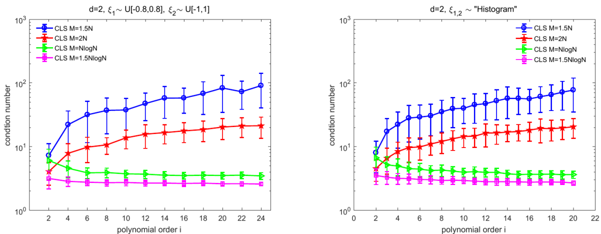
图 23 左：2 维均匀输入（纯连续分布）的条件数：对数线性采样率（log-linear）平稳。右：直方图原始数据的条件数：数据只有一份 经验直方图时，构基与采样照常工作，条件数行为与合成分布一致。
