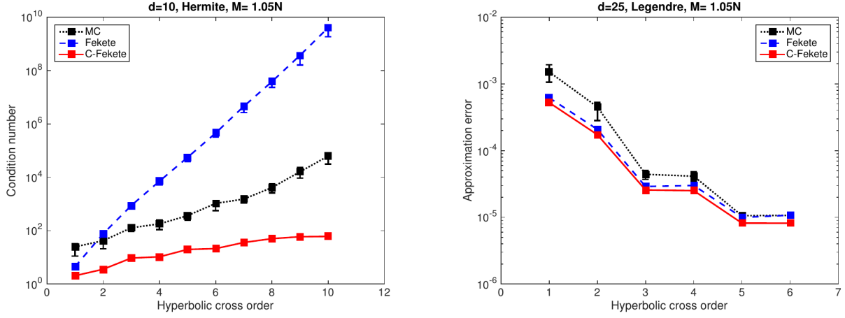
图 10 左: d = 10 Hermite (HC 指标集) 的条件数: 三种点集的差距比 Legendre 情形小, 与第一篇“无界域 L 因子较大、各方法差距缩小”的观察一致。右: 扩散方程 d = 25 (HC 指标集) 的 QoI 逼近误差: 高维下 CFP 与 AFP 相当、远好于 MC, 验证确定性点集可以走到 d = 25 。
