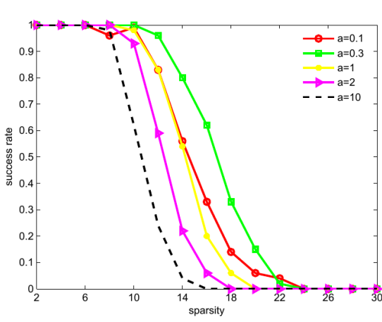
图 18 左：恢复率随 a 的扫描 ( d = 2, k = 20, N = 231, M = 45 ): a = 0.3 附近最优, 过小 (过近 \ell_0 , DCA 易陷局部) 与过大 (退化为 \ell_1 ) 都变差。右：随机 KdV 方程的相对 RMSE: TL1 与 \ell_{1-2} 、 \ell_1 的对比, TL1 在两个维数上都最低。
