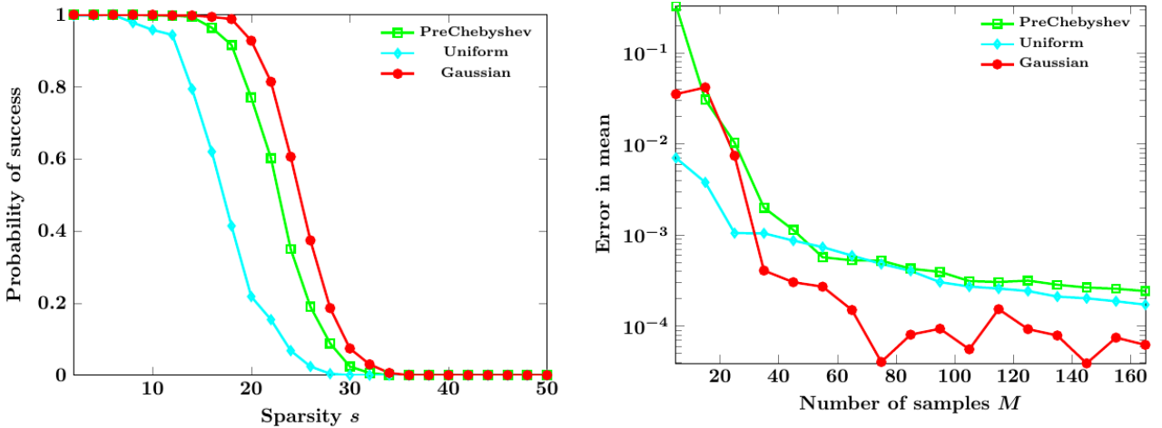
图 4 左: M = 85 时稀疏 Legendre 展开的恢复概率 ( d = 2 与 d = 10 ), Gauss 网格子采样 (Gaussian) 与其他采样策略的对比, 低维高维都不劣或更优。右: d = 3 随机椭圆 PDE 的均值 \ell_2 误差, Gauss 子采样与高精度 稀疏网格参考解一致。
