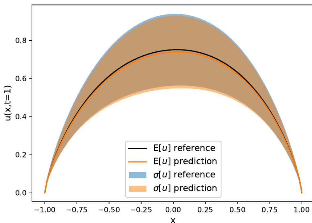
图 30 19 维随机分数阶反应扩散、噪声初值（30 个传感器加 \sigma = 0.1 噪声）下的均值与方差预测（误差棒为参考解的波动）。模态分解 + GL 离散的组合没有放大观测噪声。
