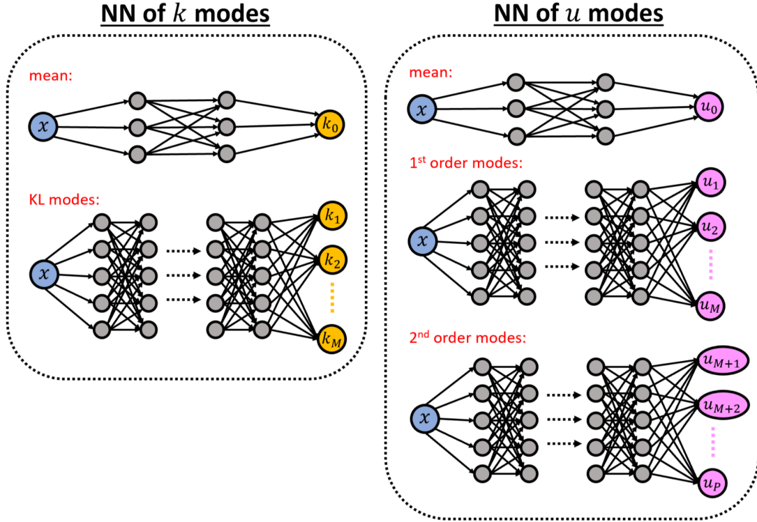
图 6 模态网络的分组结构 (论文 1809.08327)。 k 的各阶模态与 u 的各阶模态 分别分组输出。分组的依据是模态振幅的尺度：把尺度相近的模态放进同一个网络，避免优化时大尺度模态淹没小尺度模态。
