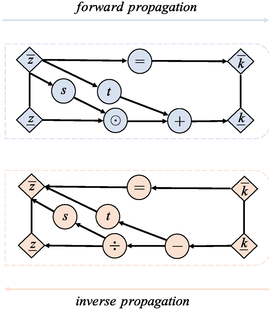
图 17 RealNVP 耦合块与多层 flow (论文 2108.12956)。每块只动一半变量，缩放因子 \exp(s) 与平移 t 由另一半通过神经网络算出。因为被动的部分不经过任何网络，雅可比是三角阵，行列式只在对角线上。多层交替堆叠后，简单高斯被逐块塑造成任意复杂的目标分布。
