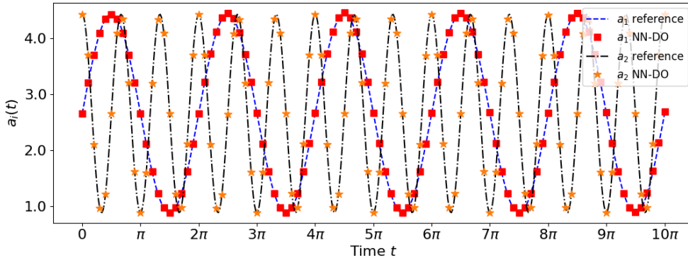
图 11 特征值交叉的实拍 (论文 1905.01205, 随机 Burgers 方程长时间积分)。图中 a_1(t) 与 a_2(t) 的曲线在时域内多次相撞: 方差第一的模态和方差第二的模态互换身份。经典 BO 方法在每个交叉点都需要特殊处理, NN 版本要绕开的就是这个。
