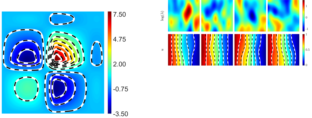
图 32 左: 52 维随机 Helmholtz 方程的解均值场 ( D_\zeta = 52 , D_x = 2 ): 生成模型学 52 维系数分布, 基网络学空间结构。右: 2 维 Darcy 流: 渗透率 \lambda 与解 u 各配一组基网络, u 均值误差 1.01%。
