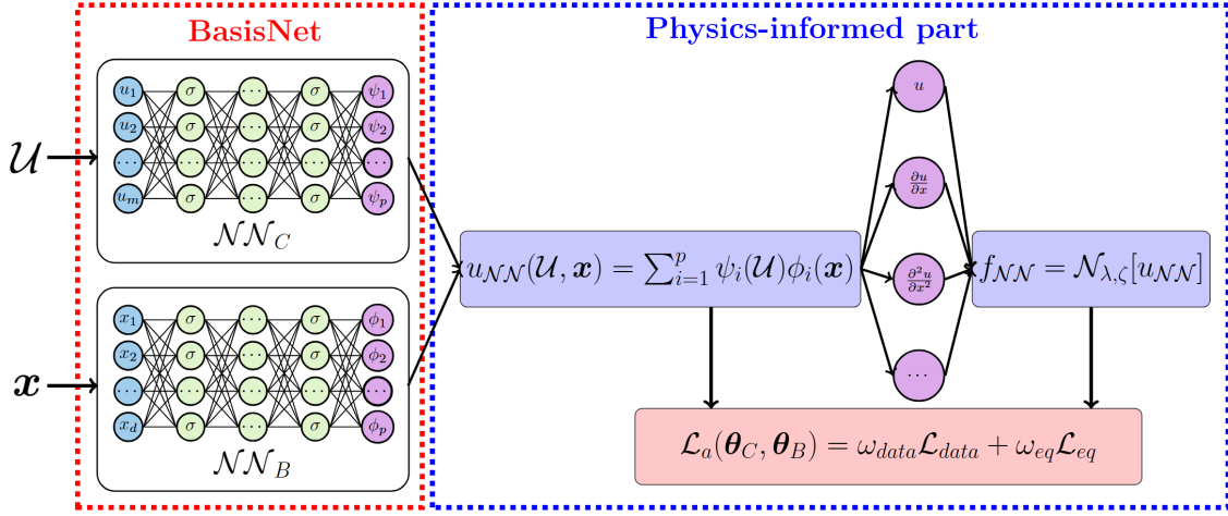
图 27 PI-BasisNet 的结构（论文 2503.18012）。输入函数 f/b （随机源项或边界）先被总结成一个表示 \mathcal{U} （随机传感器点加 PCA 主成分，或摘要网络），系数网络 \mathcal{N}_C 从 \mathcal{U} 输出 p 个系数 \psi_i ，基网络 \mathcal{N}_B 输出 p 个空间基函数 \varphi_i ，解是二者的内积。物理残差损失作用在重构出的解上。
