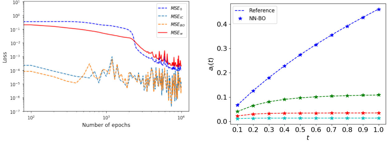
图 16 左：各损失分量的训练曲线：弱形式、约束、初值边界各自收敛，权重设计（约束项放大）的依据是它们的相对量级。右：反问题中各阶振幅 a_i 的学习轨迹：反应系数识别（真值 0.5 与 0.3）在振幅结构上留下可读的印记。
