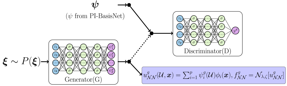
图 28 PI-GeM 的两阶段流程 (论文 2503.18012)。上半: PI-BasisNet 用数据与物理残差训练出基函数与对应的确定性系数; 下半: WGAN-GP 在系数集上学分布, 生成器输出的系数向量配上基函数即生成完整的随机场样本。
