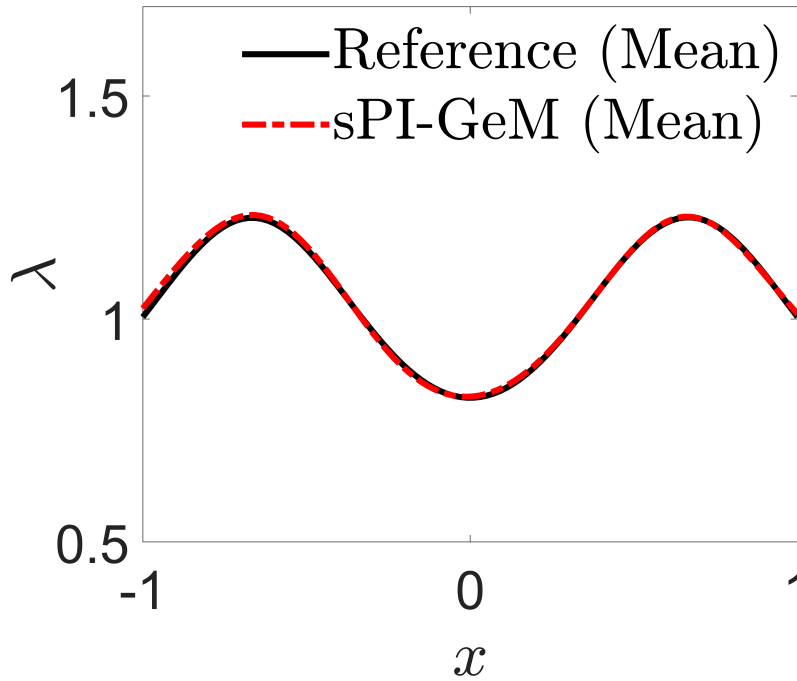
图 33 一维随机椭圆反问题: 系数网络输出拆成 u 与 \lambda 两半 (共享潜表示), 同时重构解与渗透率场。 \lambda 均值误差 0.56%、标准差误差 2.40%。
