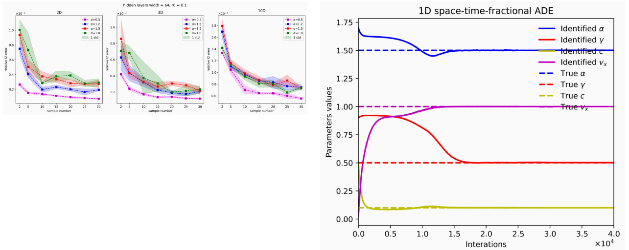
图 22 左: 相对 L^2 误差随 MC 样本数 m 的变化 (2D/3D/10D, 论文 2203.08501)。误差在约 10^{-3} 处饱和, 对 m 不敏感, 10 维与 2 维行为一致。右: 反问题中四个参数 ( \alpha, \gamma, c, v ) 的识别随训练的收敛, 真值以虚线标出。
