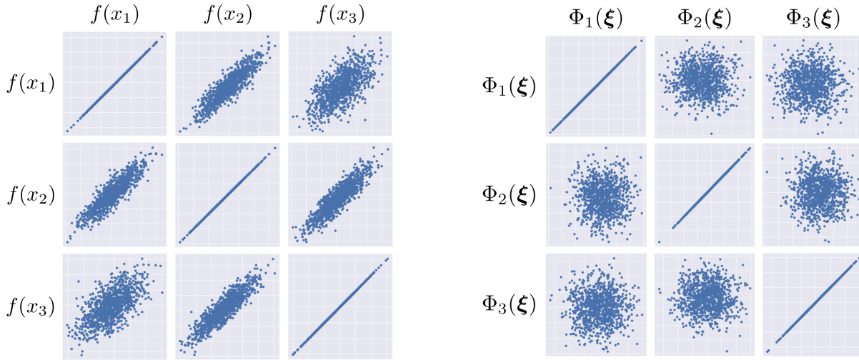
图 8 左：传感器数据中隐变量的样本相关矩阵：非对角元非零，变量之间相关。右：aPC 基函数在数据点上的相关矩阵：严格对角。正交化把相关的输入变成了不相关的特征，这是展开系数可以逐个计算的根据。
