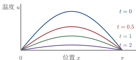
图 1 热方程 u_t = u_{xx} ( D = 1 ) 在初始条件 u(x, 0) = \sin x 、两端零温边界条件下的解，四个时刻。空间形状不变，幅度按 e^{-t} 衰减：初始条件决定“衰减哪个形状”，边界条件决定“热量从哪里流走”。
