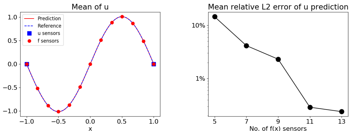
图 9 左：解的均值场预测与参考（Monte Carlo 128 条）对照。右：误差随传感器数量的衰减：信息融合的效果随数据量单调改善，一阶模态在 13 个源项传感器下已够用。
