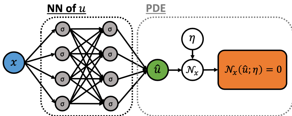
图 4 PINN 的基本构造 (论文 1809.08327 的示意图)。同一个输入 x 喂给两个网络：解网络 \hat{u}(x; \theta) 和残差网络 \hat{f}(x; \theta, \eta) 。残差网络没有自己的输出层，它把 \hat{u} 代进方程算出残差；自动微分负责求出方程里需要的各阶导数。损失函数由“数据失配”和“残差”两部分组成。
