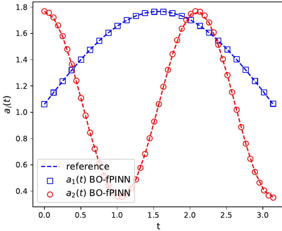
图 25 特征值交叉基准中的振幅演化 (论文 2303.10913)。 a_1(t) 与 a_2(t) 多次相撞又分开；经典 BO 的闭式解在每次相撞时分母为零，BO-fPINN 的隐式约束损失在整个时域上光滑。
