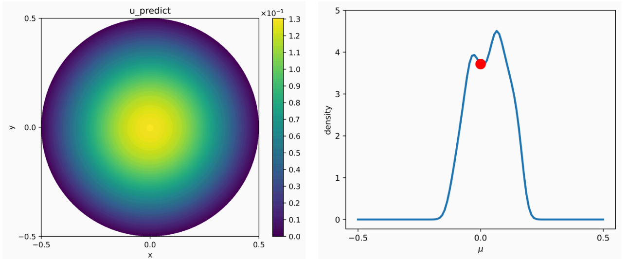
图 24 左：随机参数分数阶扩散方程 ( d = 5 ) 的代理预测与误差。右：ABC 筛选得到的 \mu 后验分布：真值落在后验峰附近，验证代理 + ABC 组合可以做完整的不确定性量化。
