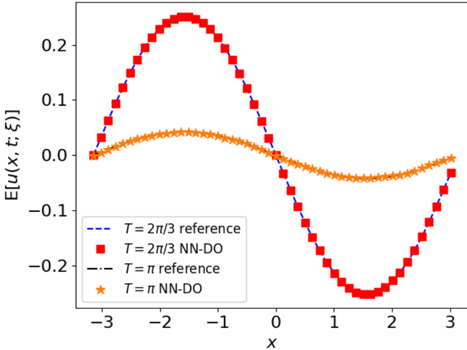
图 14 平流方程的均值场：NN-DO 的 \bar{u}_{nn} （点）与闭式 -\sin x \cdot e^{-\sigma^2 t^2/2} （线）对照，衰减形状一致。
