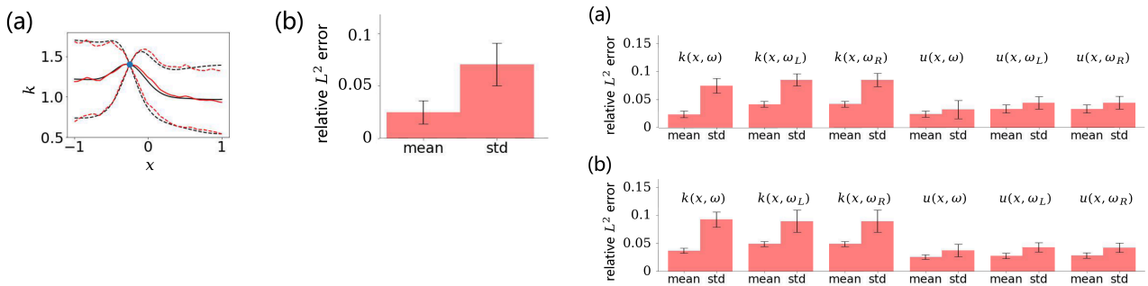
图 20 左：单点测量的后验推断：后验均值与方差包住真值，验证闭式后验公式。右：一维随机椭圆方程反向与混合问题的误差 ( N_k = 1 或 3 个 k 传感器 + 若干 u 传感器)，与蒙特卡洛参考同量级。
