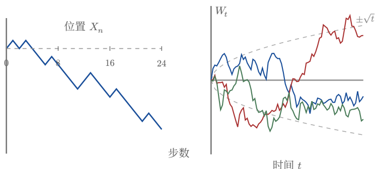
图 2 左：24 步随机游走，每步位移 \pm 1 ，折线是位置随步数的变化。右：步长与时间间隔同时缩小后的三条布朗运动路径（虚线为 \pm 一个标准差 \sqrt{t} ）。两条包络线张开的宽度随 \sqrt{t} 增长，对应方差随 t 线性增长。
