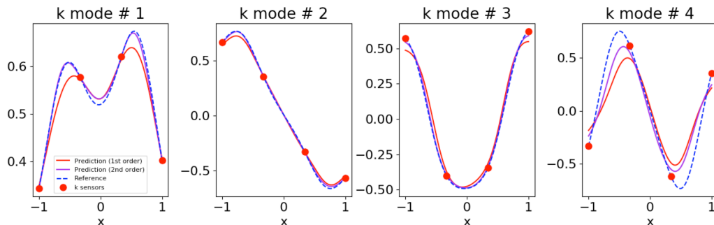
图 10 反向问题识别出的 k 各阶模态（二阶 aPC）：均值模态 k_0 平滑，一阶模态承载主要的空间变化，二阶模态幅度小但非零，它修正的是方差层面的结构。
