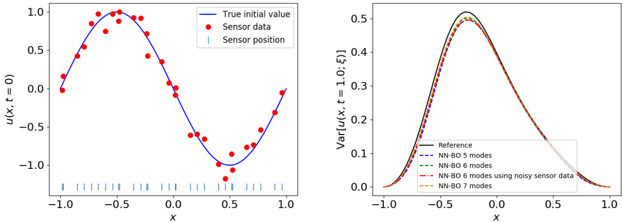
图 15 左：噪声初值（30 个传感器读数加 \sigma = 0.1 高斯噪声）对末端预测几乎无影响：模态分解天然滤掉了高频观测噪声。右：19 维扩散反应方程的方差场：6 个 BO 模态捕捉大部分随机能量。
