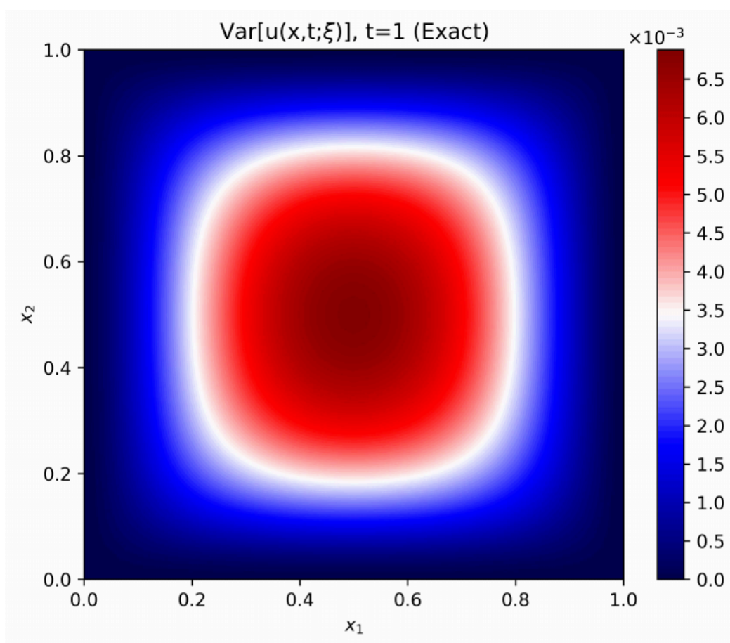
图 31 二维双 Riesz 随机分数阶反应扩散的方差场（ \alpha = 1.8 ，随机系数 + KL 型随机强迫，QMC+GL 参考解）：方差的空间结构与参考解一致，长时间积分按时域分段训练。
