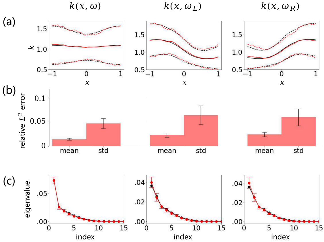
图 19 混合双模态非高斯场（一半概率加正弦、一半概率减正弦）：生成路径的均值、标准差与协方差谱（论文 2108.12956）。按两个条件模态分别对比，双峰结构被 flow 精确表达。
