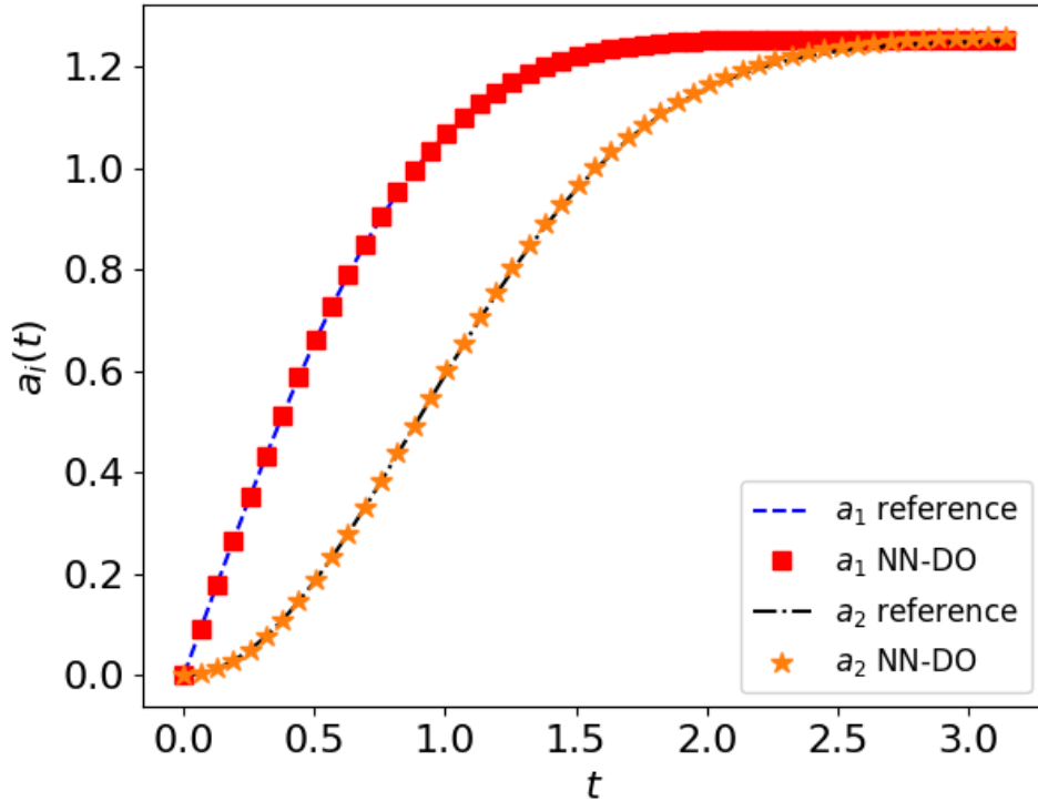
图 13 随机平流方程的 NN-DO 结果（论文 1905.01205）。方程 u_t + \xi u_x = 0 , \xi \sim N(0, 0.8^2) ，确定性初值 u(x, 0) = -\sin x 。振幅 a_i(t) 从零开始增长：随机性由随机平流速度逐步注入。该例有精确的 DO 解（如 u_1^{\text{DO}} = -\frac{1}{\sqrt{\pi}} \cos x , Y_1^{\text{DO}} = -\sqrt{\pi} \sin(\xi t) ），NN-DO 各分量与精确解的相对 L^2 误差在 2% 以内。
