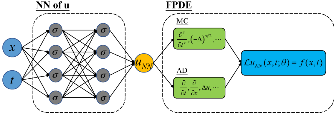
图 21 MC-PINN 总框架 (论文 2203.08501)。对每个训练点: 随机采样方向 \xi 与半径 r (内段与外段各一组分布), 在 x \pm r\xi 处评估网络, 构造分数阶算子的无偏估计; 两次独立估计相乘构成物理损失。与 fPINN 的 GL 求积相比, 评估次数从 q^d \times L 降到 8m + 1 , 与维数几乎无关。
