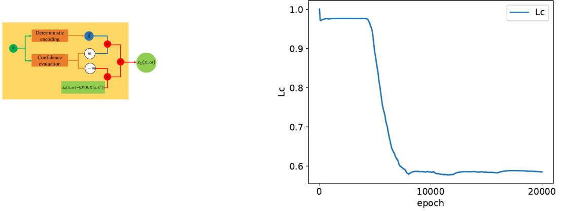
图 31 LVM-GP 的编码器结构与先验自适应 (论文 2507.22493)。左: 确定性特征 \bar{z} 、置信门 m 与 GP 先验 z_0 的插值结构 (与 IB-UQ 同构, 先验换成带空间相关的 GP)。右: GP 核长度尺度的训练曲线: 从初始 1.0 自适应收敛到 0.58, 先验自己学到了数据的相关长度。
