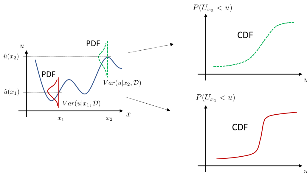
图 8 从样本到校准判据的一步（综述 2201.07766 附录）：后验样本给出预测 PDF，积分成 CDF，再按名义概率读分位数与覆盖率。RMSCE 就是在最后这一步上量“名义概率与经验覆盖率的差”。
