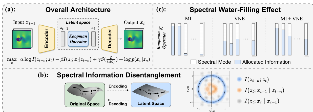
图 5 论文 Figure 1。(a) 整体架构与拉格朗日量；(b) 信息解耦：把原空间到潜在空间的映射与三类信息放到同一个复平面上，蓝色环对应 I(z_{t-n}; z_t) （单位圆上的相干模式），橙色中心对应 I(z_t; x_{t-1} | z_{t-n}) （圆内的耗散模式），灰色散点对应 I(z_t; x_t | x_{t-1}) （无谱对应）；(c) 谱注水效应：MI（只有互信息）会把信息堆到少数几个模式上，VNE（只有熵）会均匀铺开，只有 MI+VNE 同时作用才得到既有侧重又不坍缩的分配。
