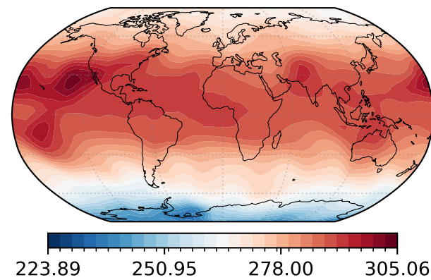
KAE
