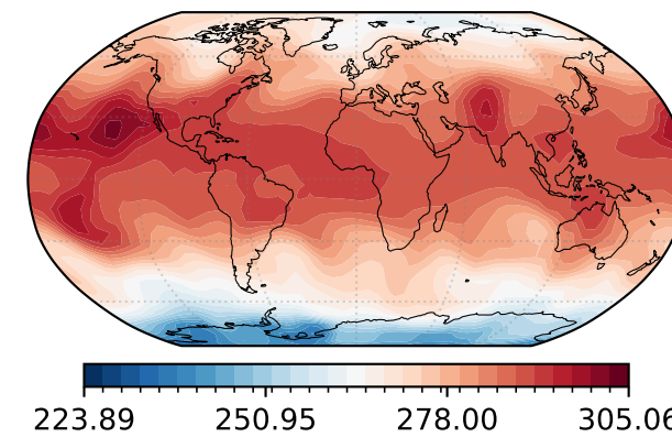
Ours
