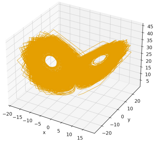
Lorenz 63
