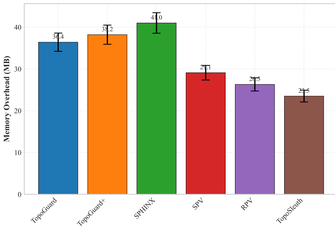
(d) Memory Overhead Comparison
