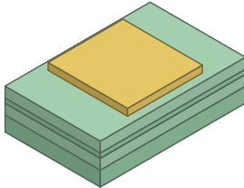
(b) AlGaAs/GaAs DH laser
