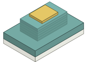
(f) InGaN/GaN micro-LED
