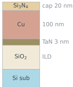
(b) Cu interconnect (BEOL)
