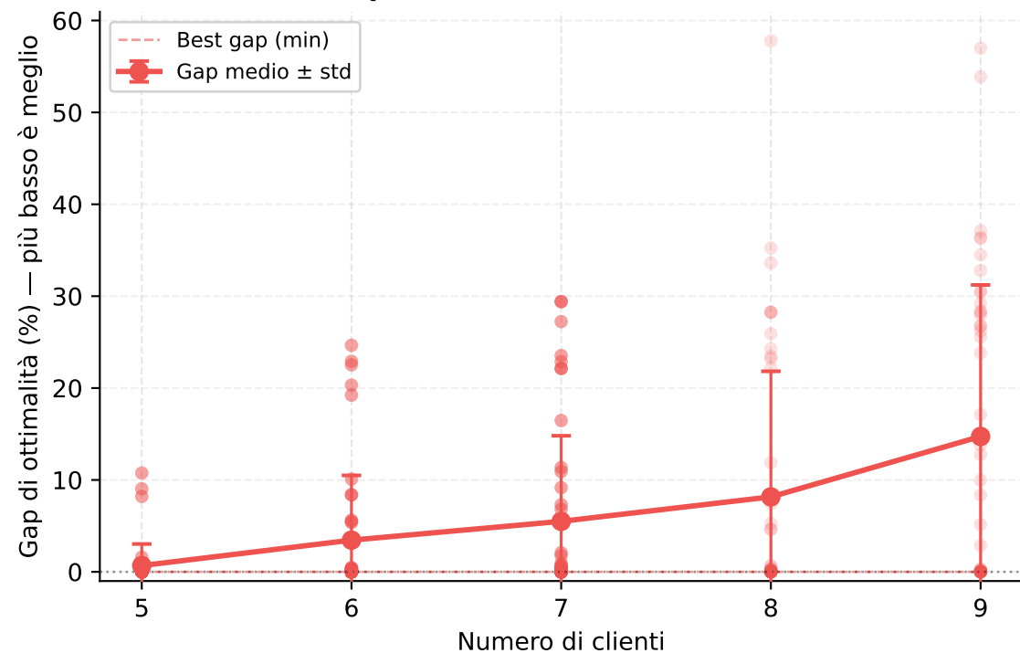
Qualità della metaeuristica
