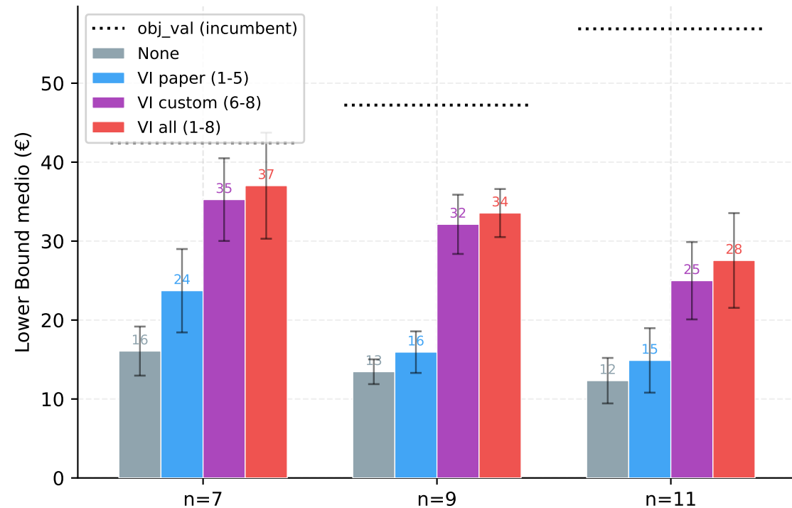
Qualità del Lower Bound
