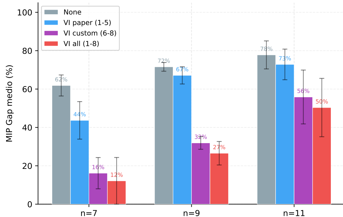
MIP Gap per configurazione VI
