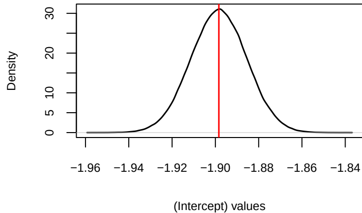
CMC posterior density of (Intercept)
