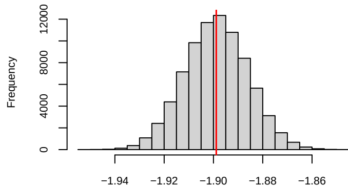
Posterior histogram of (Intercept)
