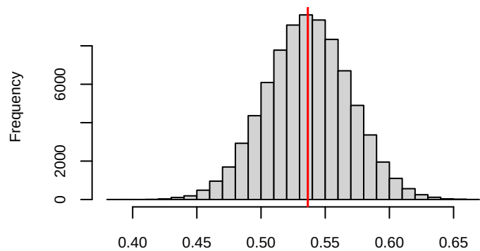
Posterior histogram of speed_limit5
