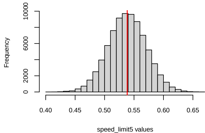
Posterior histogram of speed_limit5
