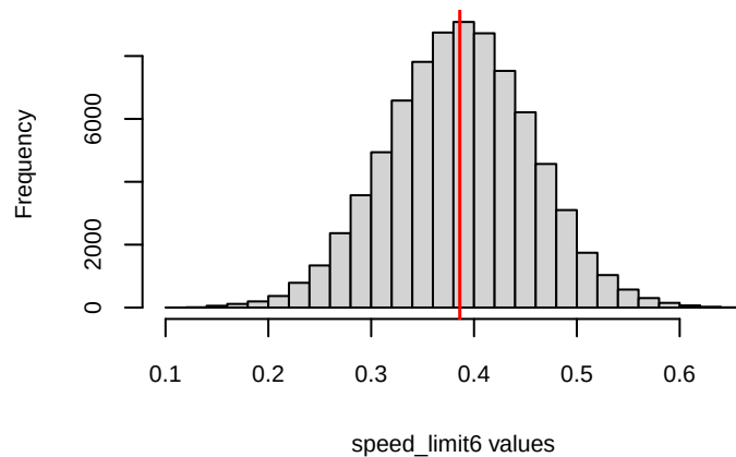
Posterior histogram of speed_limit6
